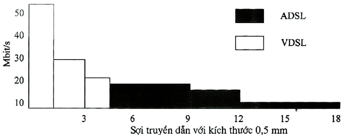
Hình 2: So sánh công nghệ VDSL với công nghệ ADSL
