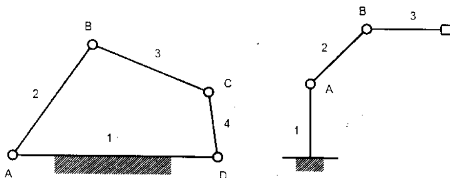
Hình 8.1: Chuỗi động học kín và chuỗi động học hở
