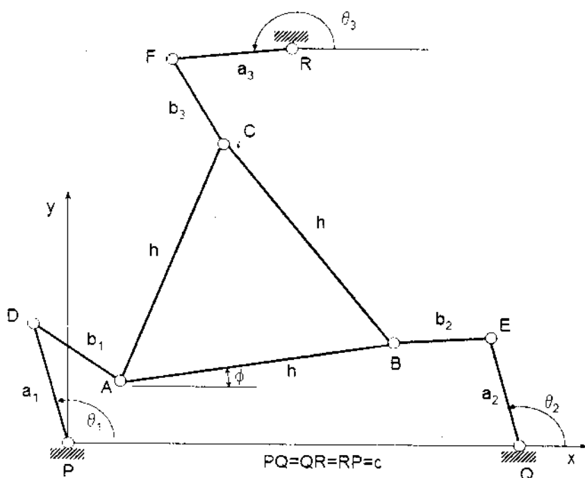
Hình 8. 4: Tay máy phẳng 3 BTĐ, RRR
