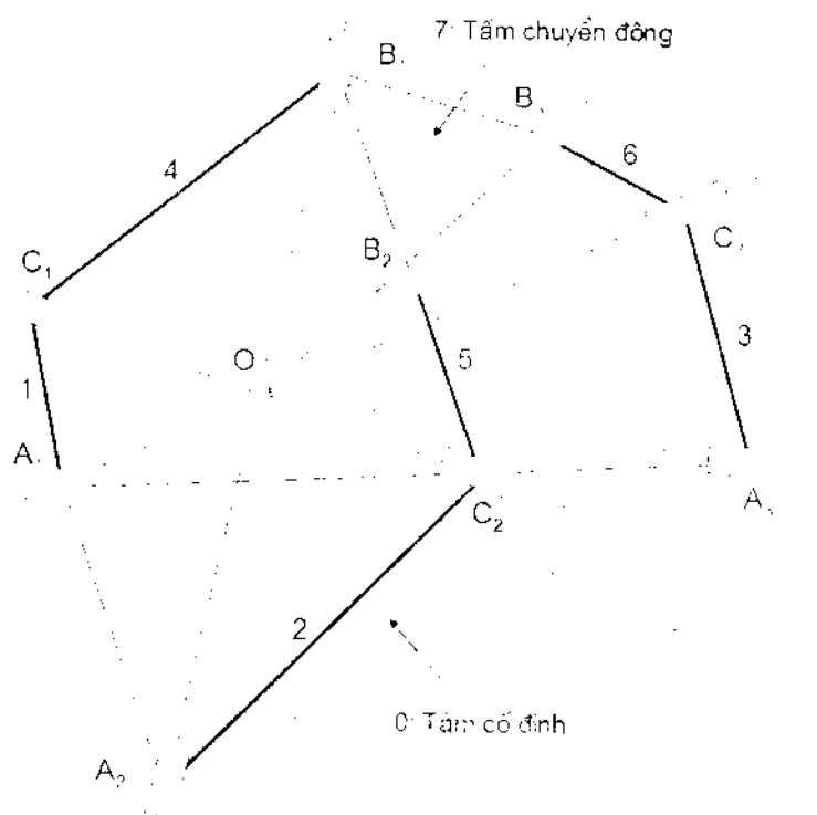
Hình 8. 5: Sơ đồ kết cấu của tay máy cân
