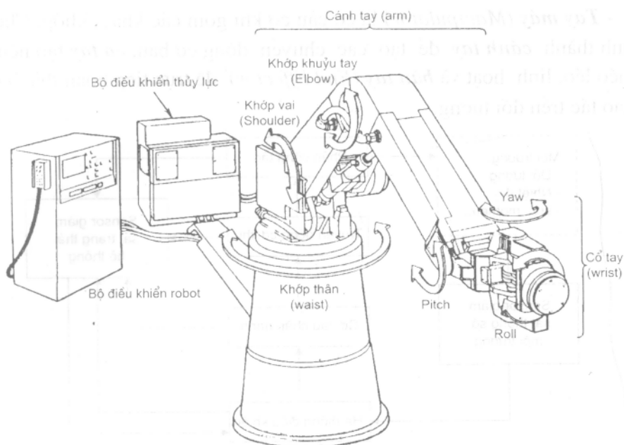
Hình 1. 2: Sơ đồ kết cấu chung của RBCN
