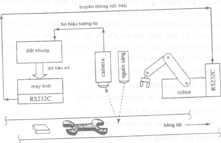
Hình 6.13: Hệ thống nhận dạng chỉ tiết
