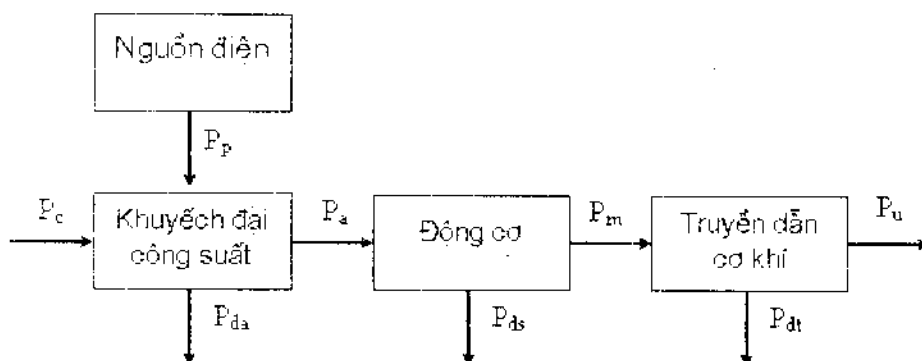
Hình 6.1: Sơ đồ hệ thống chấp hành
