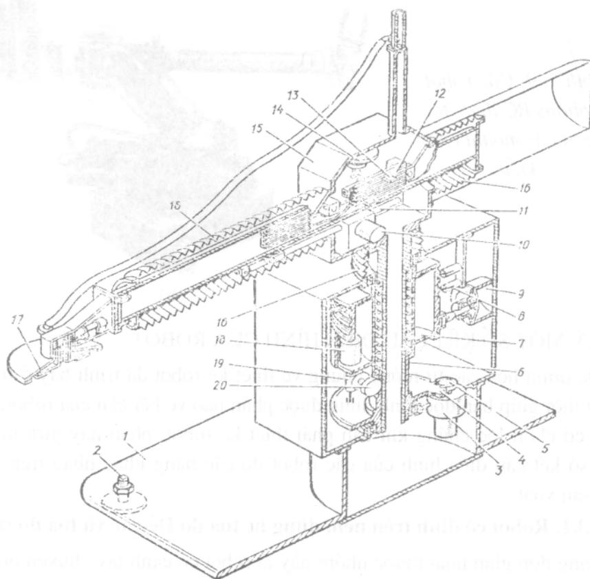
Hình 5.10: Sơ đồ động của robot MP4
