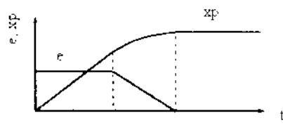
b: Điều khiển tích phân (I)
