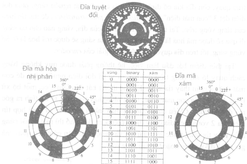
Hình 6. 8: Sơ đồ nguyên lý của thước đo vị trí tuyệt đối
