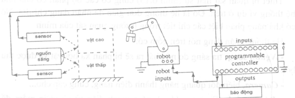
Hình 6.12: Hệ thống quan sát 2 pixel
