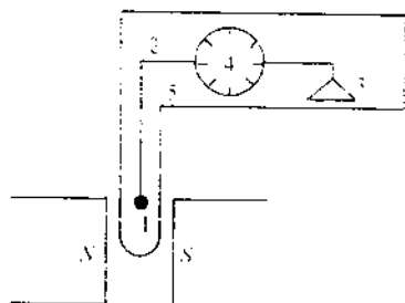
Hình 6.11. Thiết bị xác định độ cảm từ bằng phương pháp Faraday:
