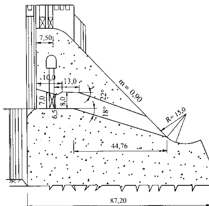
Hình 12-1. Đập tràn kết hợp xả sâu (kích thước trong hình vẽ: mét)
