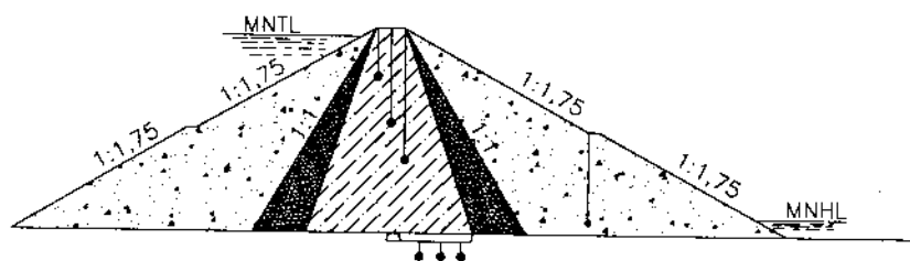
Hình 21-1. Sơ đồ bố trí ống đo áp trong thân đập và sau màng chống thấm
