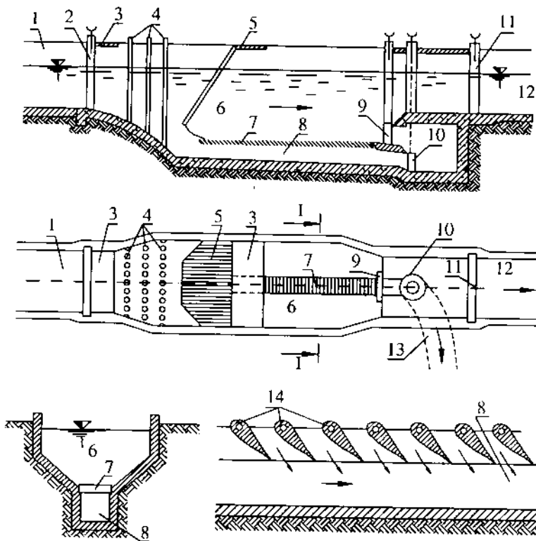
Hình 18-10: Bể lắng cát kiểu Diaphuro
