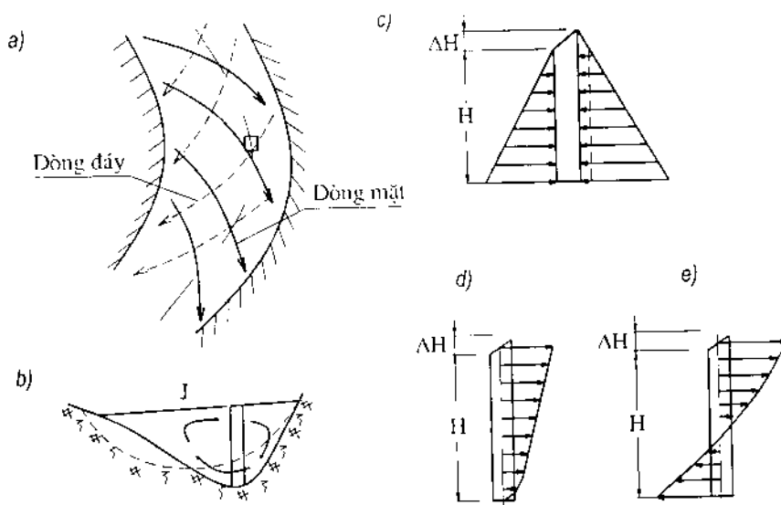
Hình 13-3. Sơ đồ dòng chảy ở đoạn sông cong
