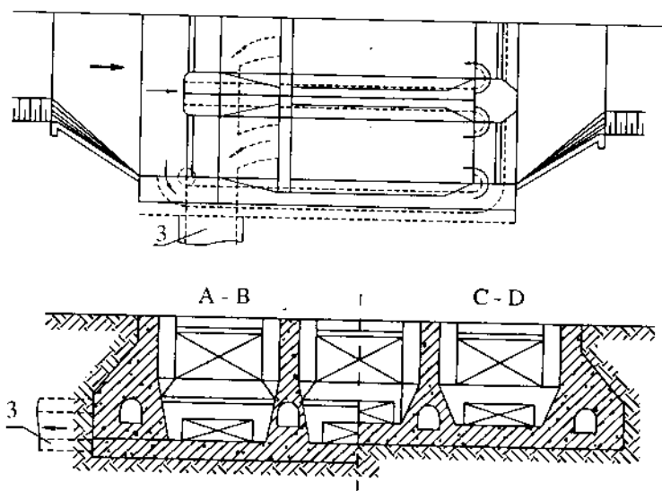
Hình 18-3. Bể lắng cát có độ dốc ngược
