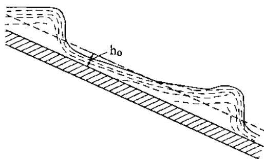
Hình 12-26. Sóng trong dốc nước
