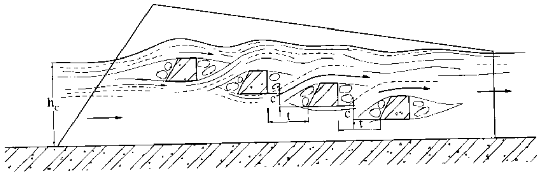
Hình 14-14. Dầm tiêu năng
