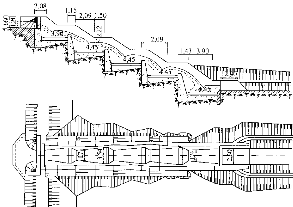
Hình 12-32. Bậc nước
