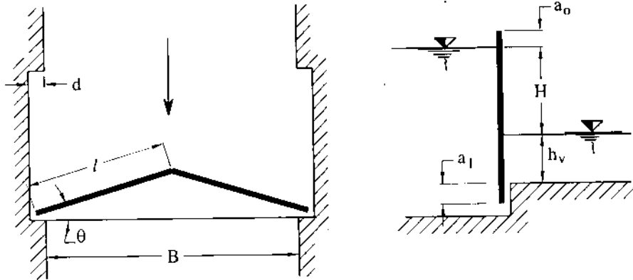
Hình 19-41: Sơ đồ kích thước van chữ V.
