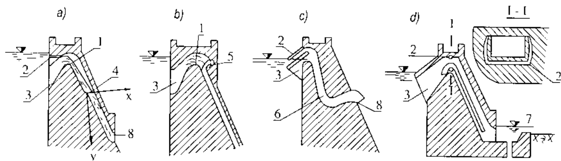
Hình 12-35. Kết cấu các bộ phận xi phòng
