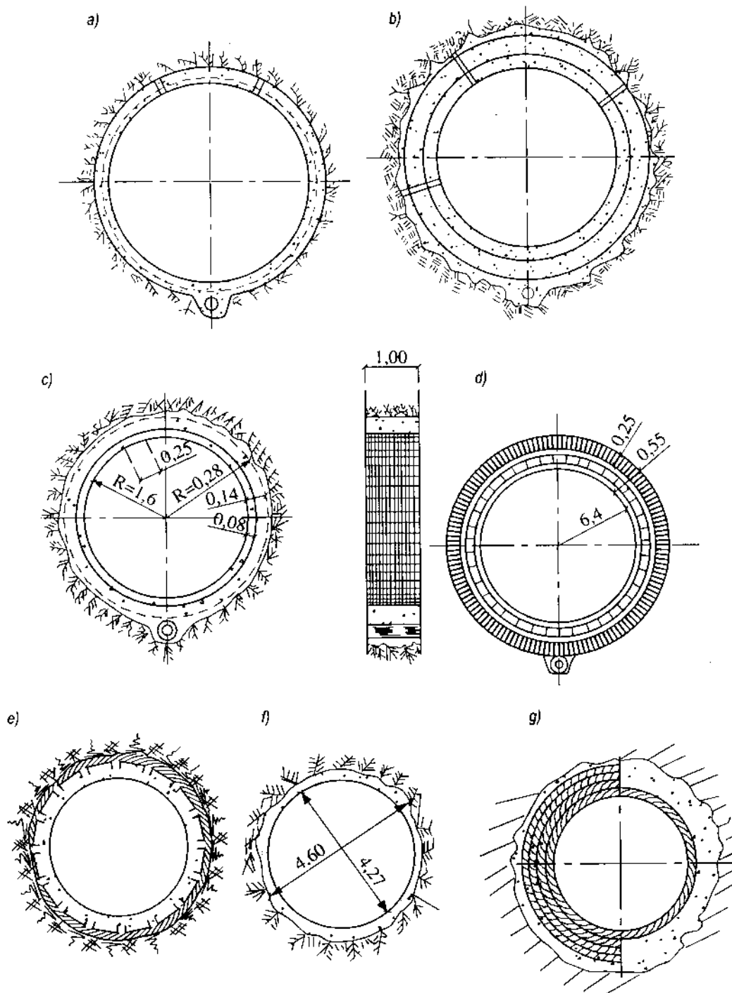
Hình 15-15. Hình thức lớp lót của đường hãm có áp
