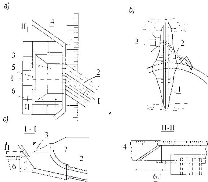
Hình 12.39. Đường tràn kiểu gáo
