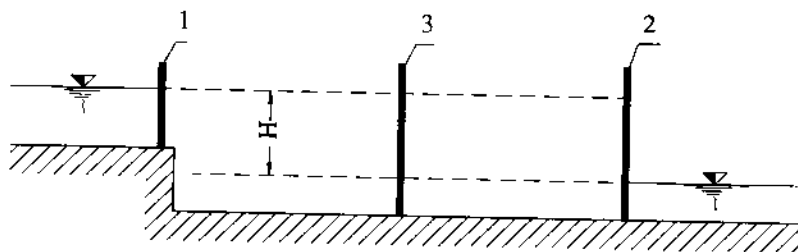
Hình 19-5: Âu thuyền đơn cấp có cửa van phụ ở giữa buồng âu.
