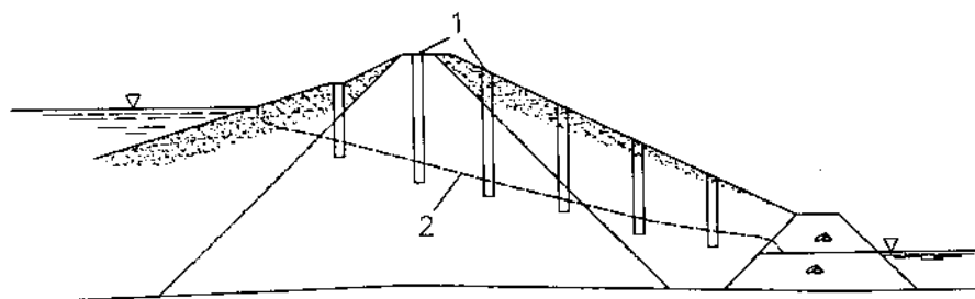
Hình 22-2. Bố trí ống đo áp trong đập đất 1. Ống đo áp; 2. Đường bão hoà
