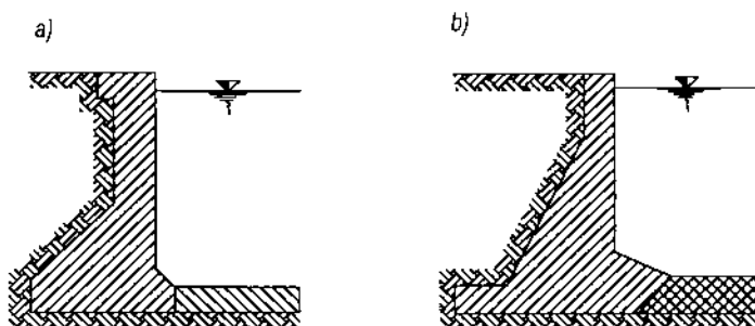
Hình 19-29 : Buồng âu không thấm nước có bản đáy tách rời.
