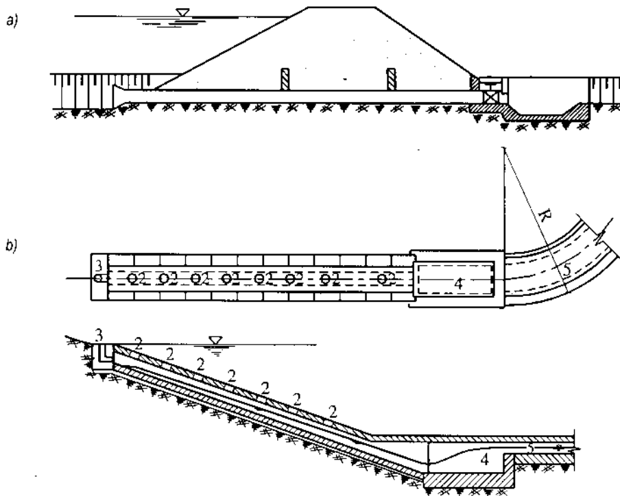
Hình 15-38. Các loại ống ngầm lấy nước
