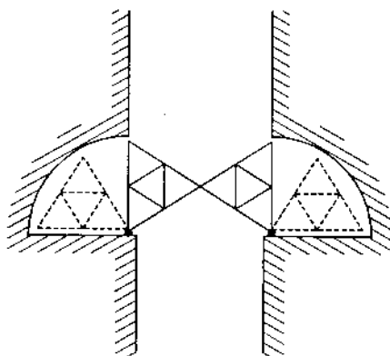
Hình 19-38 : Cửa van kiểu tam giác.
