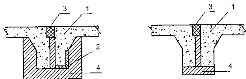
Hình 16-21. Chống thấm giữa thân máng với bộ phận cửa vào, cửa ra 1. Thân máng; 2. Bao tải tấm nhựa đường; 3. Vữa xi măng trát; 4. Bê tông lót.
