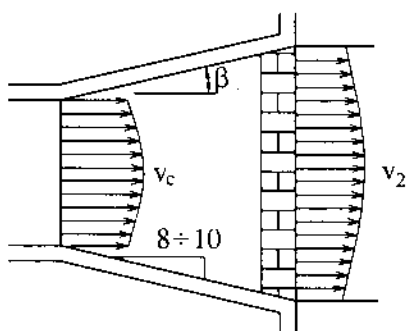
Hình 12-11. Bể tiêu năng khuếch tán
