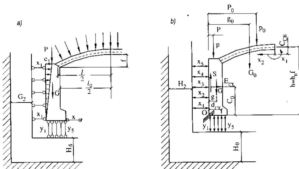
Hình 15-24. Tường bên đàn hồi a) Hình thức kết cấu; b) Sơ đồ tính toán.
