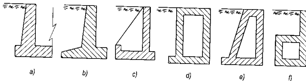
Hình 14-35. Các hình thức móng bên
