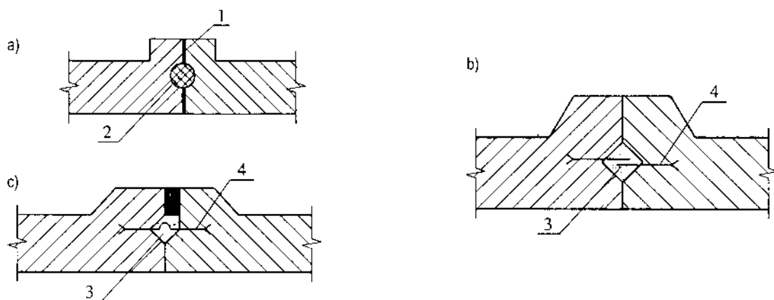
Hình 15-52. Khe nối giữa các đoạn ống
