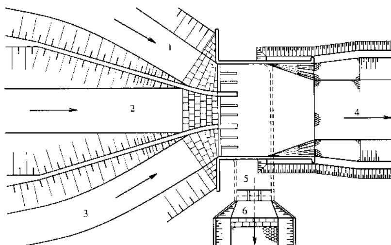
Hình 13-8. Sơ đồ bố trí lấy nước kiểu V.V. Saumian
