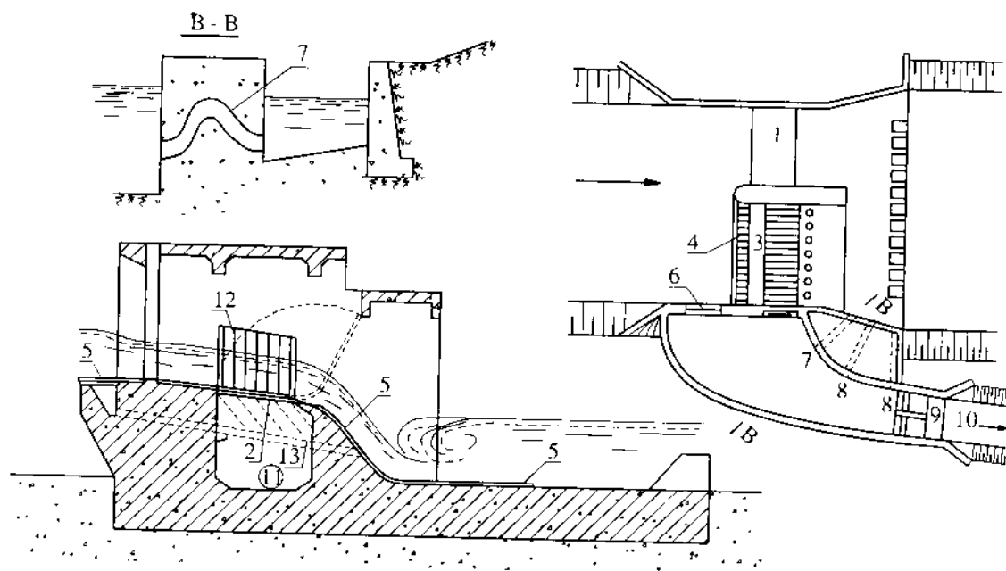
Hình 13-23: Công trình lấy nước có lưới chắn đặt ở đỉnh đập
