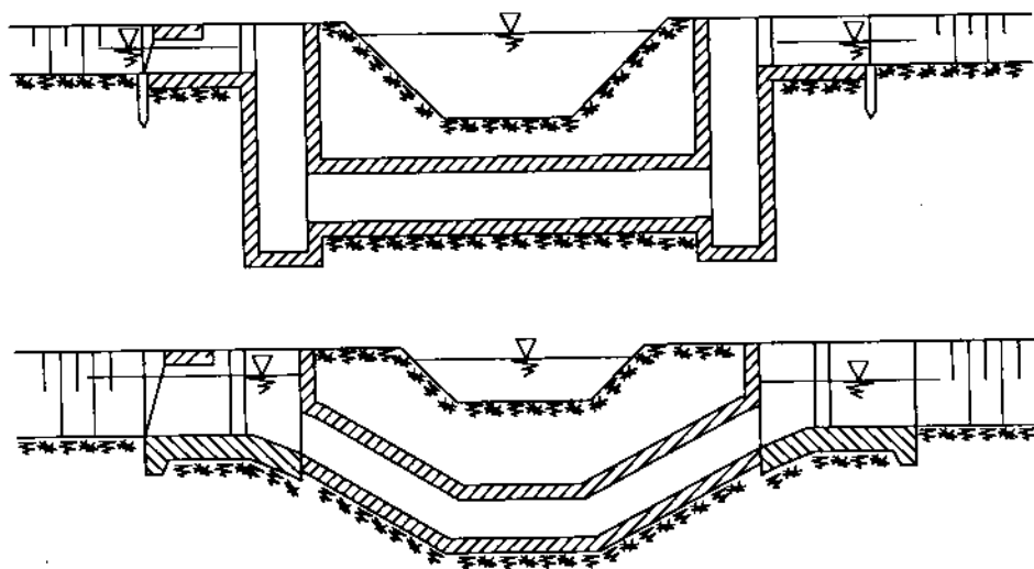
Hình 16-23. Các loại xi phông ngược:
