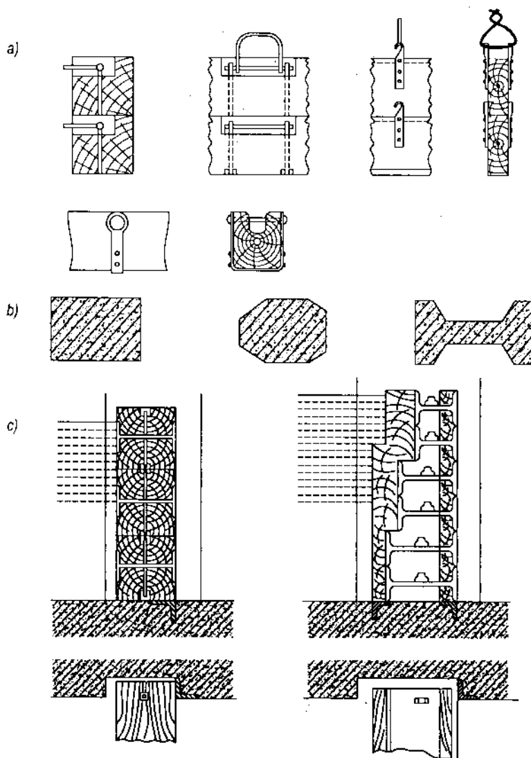
Hình 17-13. Một số hình thức phai a) Phai gỗ; b) Phai bê tông cốt thép; c) Phai thép.
