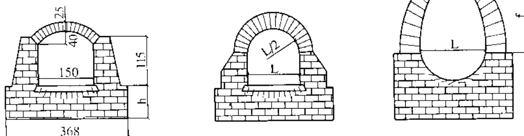
Hình 16-12. Cổng ngầm kiểu vòm
