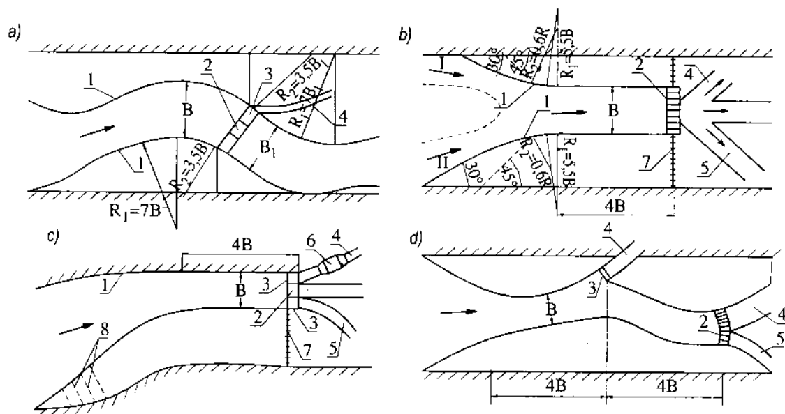
Hình 13-29. Sơ đồ chỉnh trị đoạn sông có cửa lấy nước có đập
