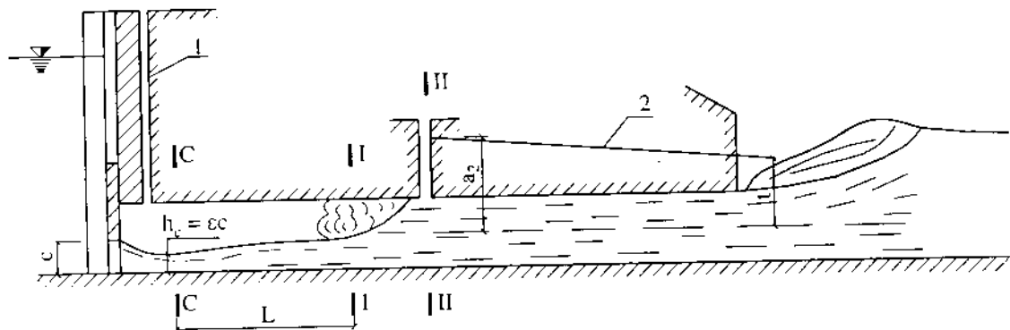
Hình 15-45. Dòng chảy sau cửa van
