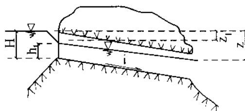
Hình 15-5. Dòng chảy ở đường hầm không áp
