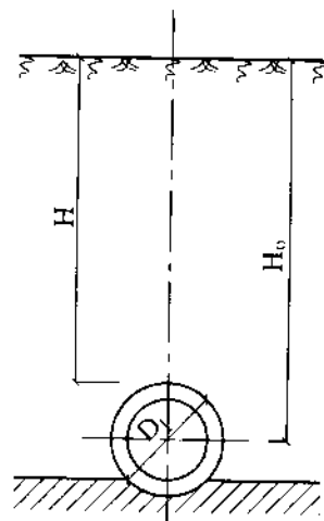
Hình 15-48. Ống đặt nổi.
