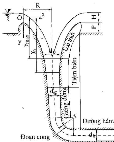
Hình 12-37. Các bộ phận của giếng tháo lũ
