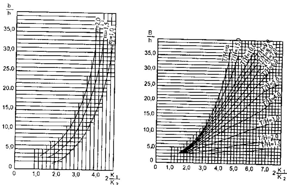
Hình 16-3. Đường cong xác định trị số 2 \frac{K_1}{K_2}
