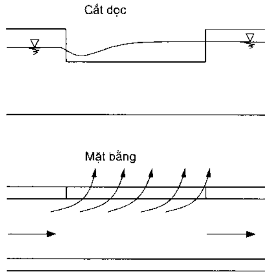
Hình 16-5. Sơ đồ tràn bên
