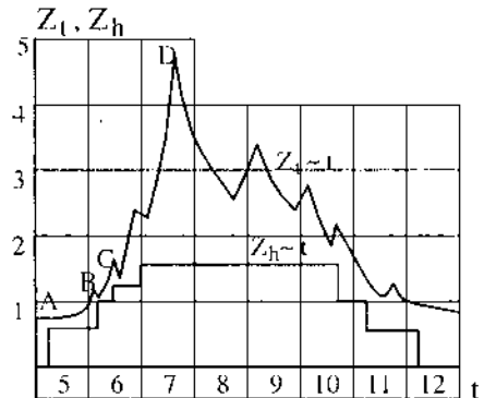
Hình 14-6. Đường quá trình mực nước thượng hạ lưu cống
