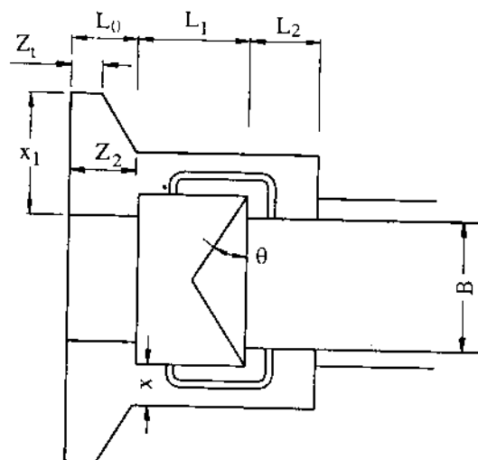
Hình 19-24: Sơ đồ đầu âu có cánh chữ V
