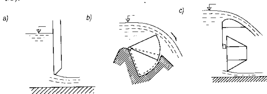
Hình 17-3. Các hình thức tháo nước qua cửa van a) Dưới đáy; b) Trên đỉnh; c) Kết hợp.
