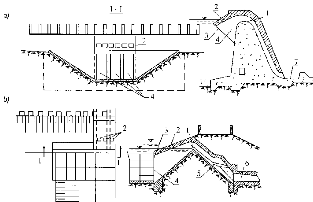
Hình 12-34. a) Xi phong tháo lũ trong đập bê tông; b) Xi phong trong đập đất.
