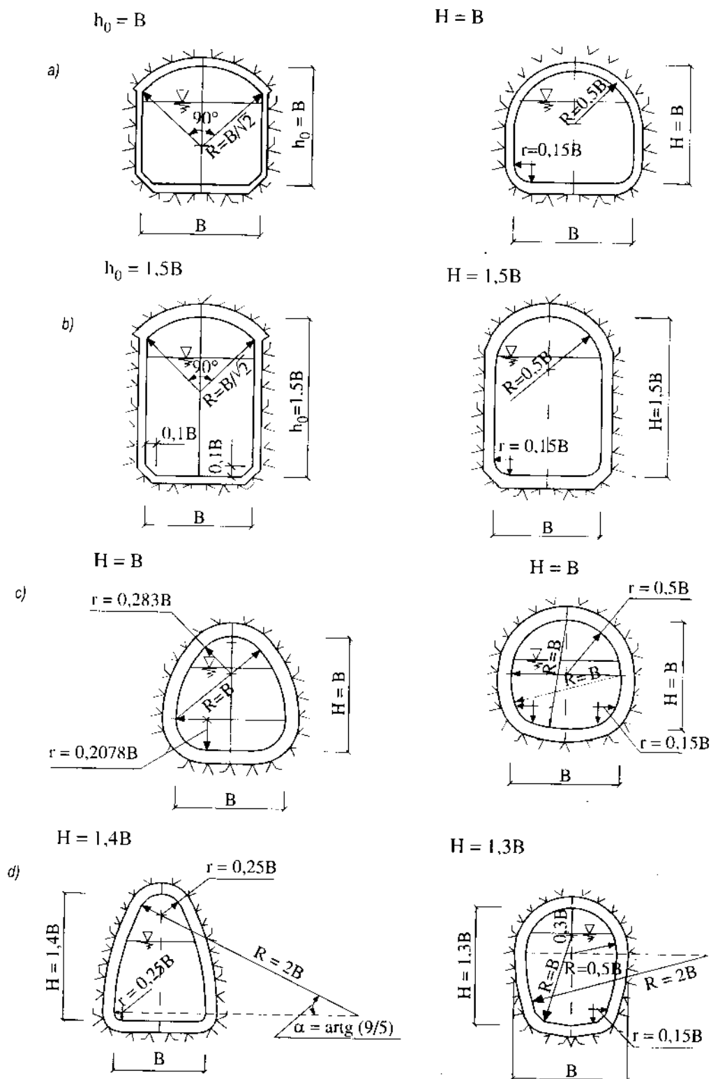
Hình 15-3. Các hình thức mặt cắt của đường hầm không áp
