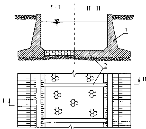
Hình 19-28: Buồng âu đáy thấm nước có đặt các thanh chống ngang. 1. Tường bên ; 2. Dầm ngang đáy.
