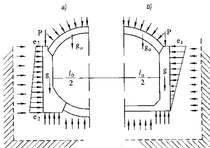
Hình 15-22. Các lực tác dụng lên tường bên
