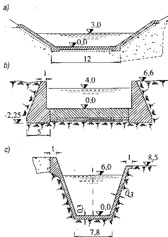
Hình 12-24. Mặt cắt ngang của dốc nước
