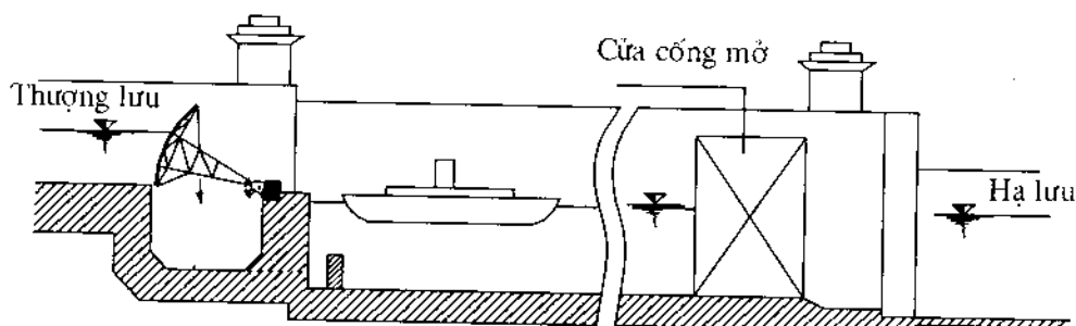
Hình 19-25: Sơ đồ âu thuyền khi mở cửa van thì hạ xuống hố ở bán đáy của đầu âu.
