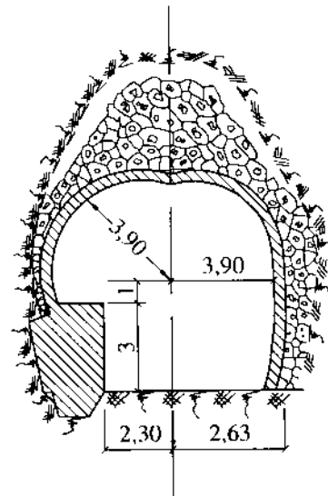
Hình 15-9. Hiện tượng đá bị sụt và hình thành vòm cân bằng tự nhiên
