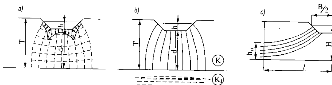
Hình 16-2. Sơ đồ nước thấm từ kênh
