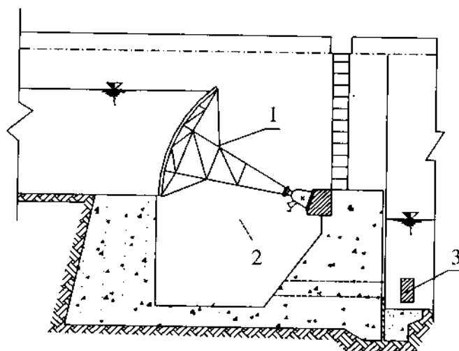
Hình 19-32 : Dẫn nước qua phía dưới cửa van cùng. 1. Van cùng; 2. Buồng tiêu năng; 3. Dầm tiêu năng.
