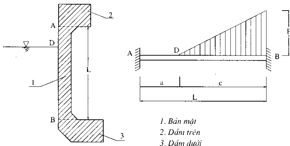
Hình 14-23. Tường ngực và sơ đồ áp lực nước tác dụng lên nó
