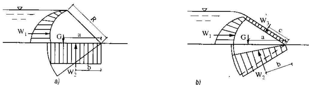
Hình 17-26. Sơ đồ lực tác dụng lên van quay
