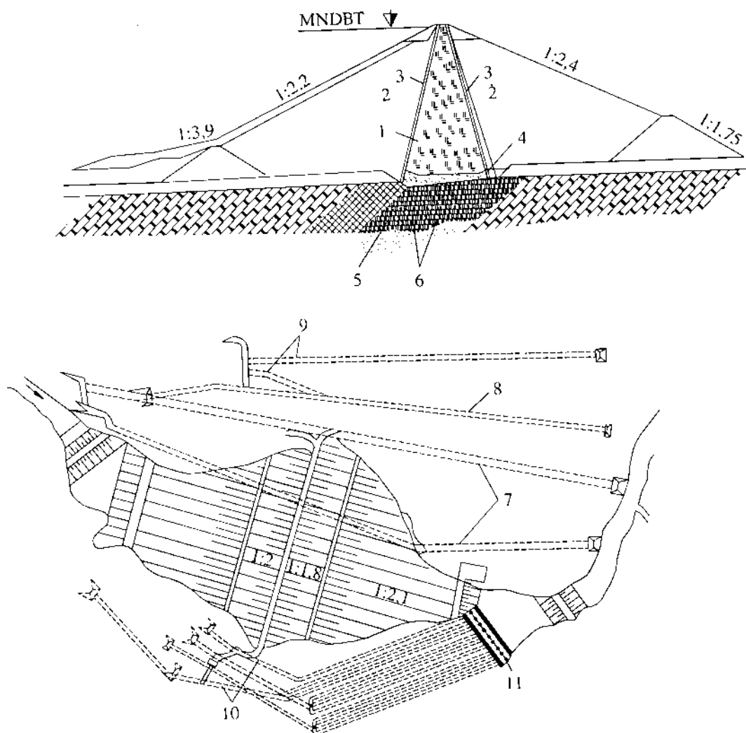
Hình 20-1. Bố trí công trình đầu mối Nuréch (Tajikixtan) có cột nước cao 1. Lõi chống thấm, 2. Các khối bên của đập đá đổ, 3. Các lớp chuyển tiếp, 4. Nút bê tông, 5, 6. Màng chống thấm, 7, 8, 9. Các đường hầm tháo lũ, 10. Đường hầm dẫn nước vào nhà máy thủy điện, 11. Nhà máy thủy điện
