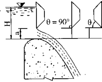
Hình 12-4. Sơ đồ nước chảy qua đập tràn có cửa van
