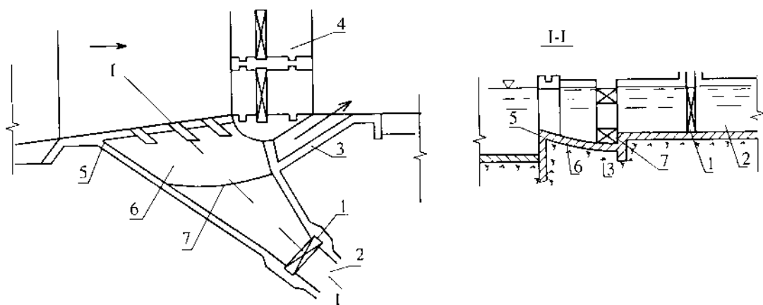
Hình 13-18: Hình thức lấy nước bên cạnh có túi chứa cát.
