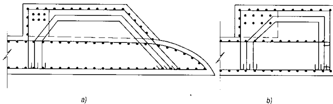
Hình 14-30. Sơ đồ bố trí cốt thép tại bệ tỷ van cùng a) Mặt cắt ngang; b) Mặt cắt đứng.
