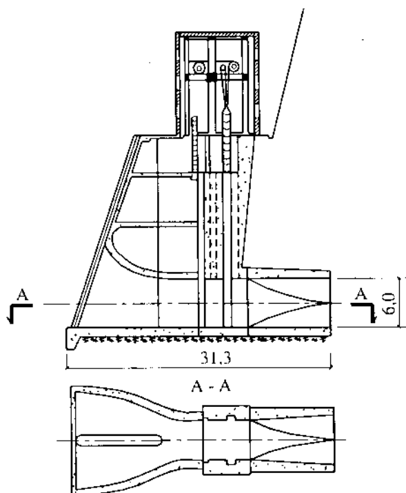
Hình 15-32. Cửa lấy nước kiểu tháp tựa bờ
