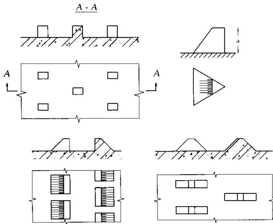
Hình 14-13. Mố tiêu năng
