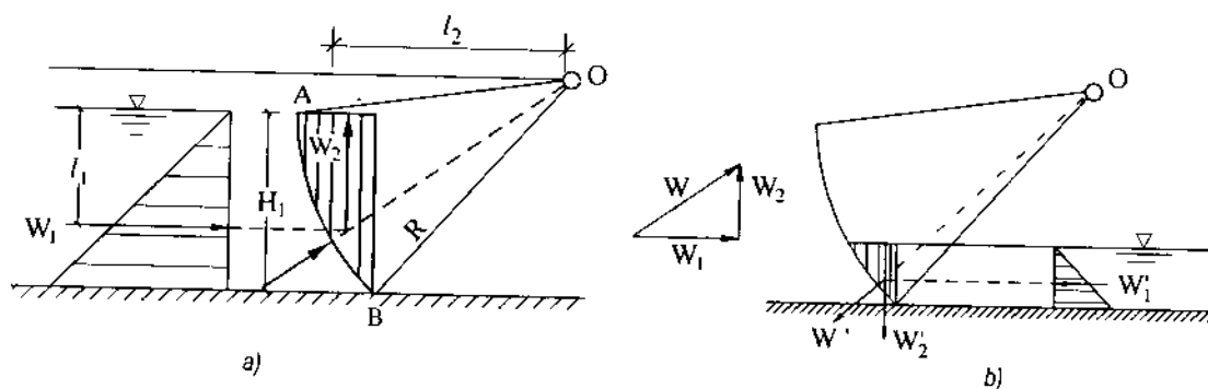
Hình 17-19. Sơ đồ áp lực nước tác dụng lên van cung
