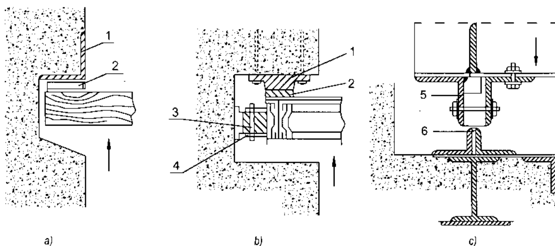
Hình 17-15. Bộ phận đỡ tựa và trượt tiếp xúc của cửa van phẳng 1. Thanh thép hình gắn vào mố trụ; 2. Thanh kim loại tỳ; 3. Thanh ray; 4. Bánh xe định hướng; 5. Gỗ ép; 6. Lớp kim loại không gỉ.
