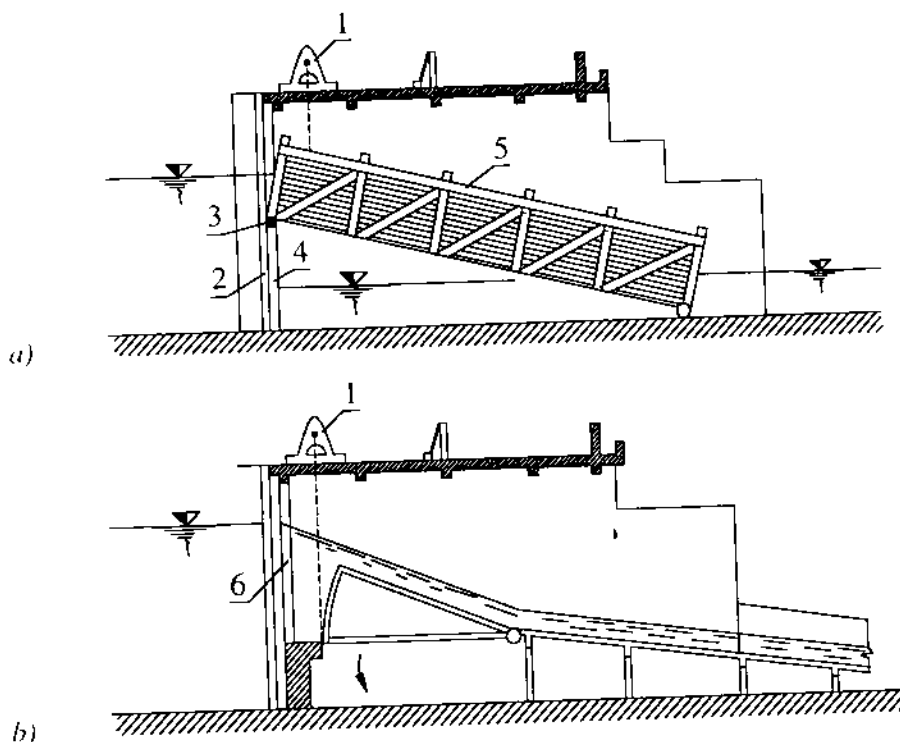
Hình 19-46: Máng kiểu di động (a) và máng có cửa van hình cung (b)
