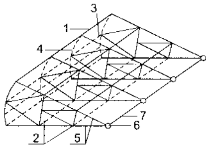
Hình 17-27. Cấu tạo cửa van hình quạt
