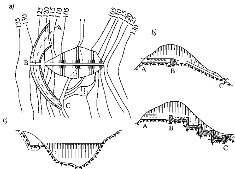
Hình 12-20. Đường tràn dọc
