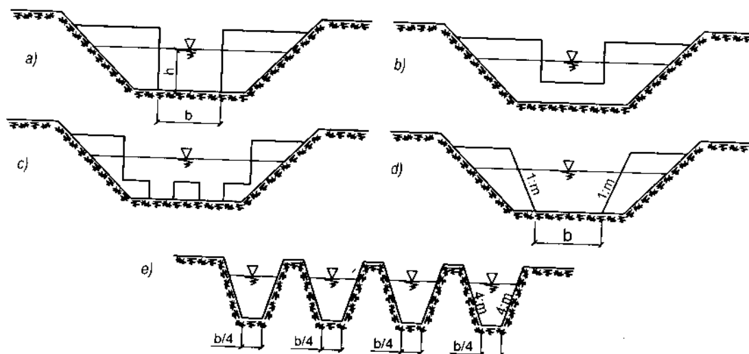
Hình 16-28. Các hình thức cửa vào của dốc nước và bậc nước
