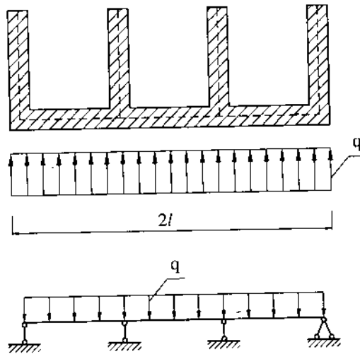
Hình 14-19. Sơ đồ tính bản đáy cống theo phương pháp dầm đảo ngược
