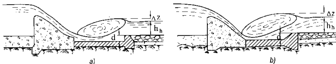
Hình 12-6. Hình thức bể tiêu năng
