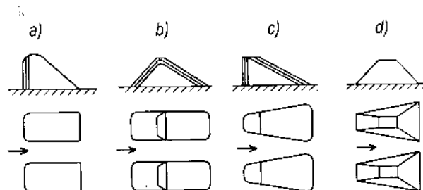
Hình 12-10. Các hình thức mố tiêu năng
