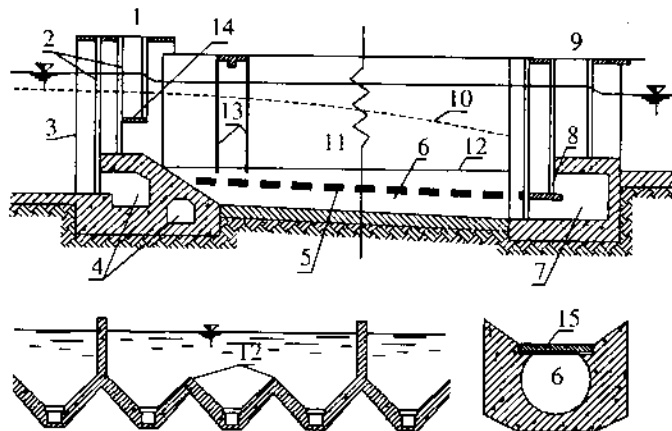
Hình 18-9 : Bể lắng cát xối rửa kiểu Zamarin
