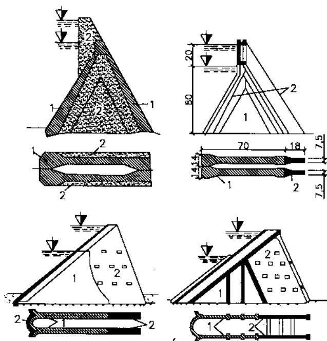
Hình 21-7. Giải pháp tôn cao và mở rộng đập bần chống 1. Khối đập cũ, 2. Khối đập tôn cao, mở rộng
