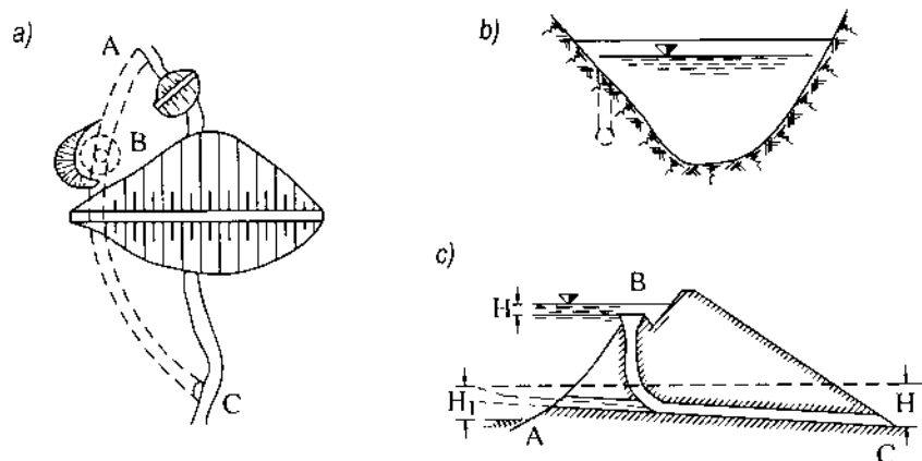
Hình 12-36. Giếng tháo lũ
