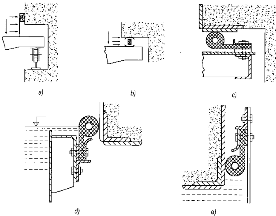
Hình 17-18. Thiết bị chắn nước bên cạnh (a, b, c) và tường ngược (d, e) a và b) Vật chắn nước bằng gỗ; c, d, e) Bằng cao su.
