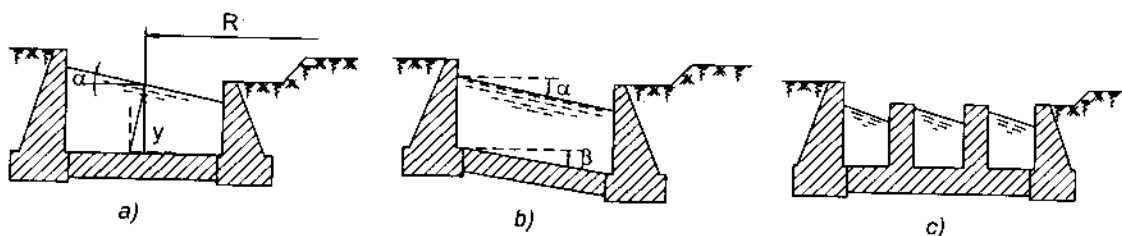
Hình 12-25. Mặt cắt ngang dốc nước tại đoạn cong
