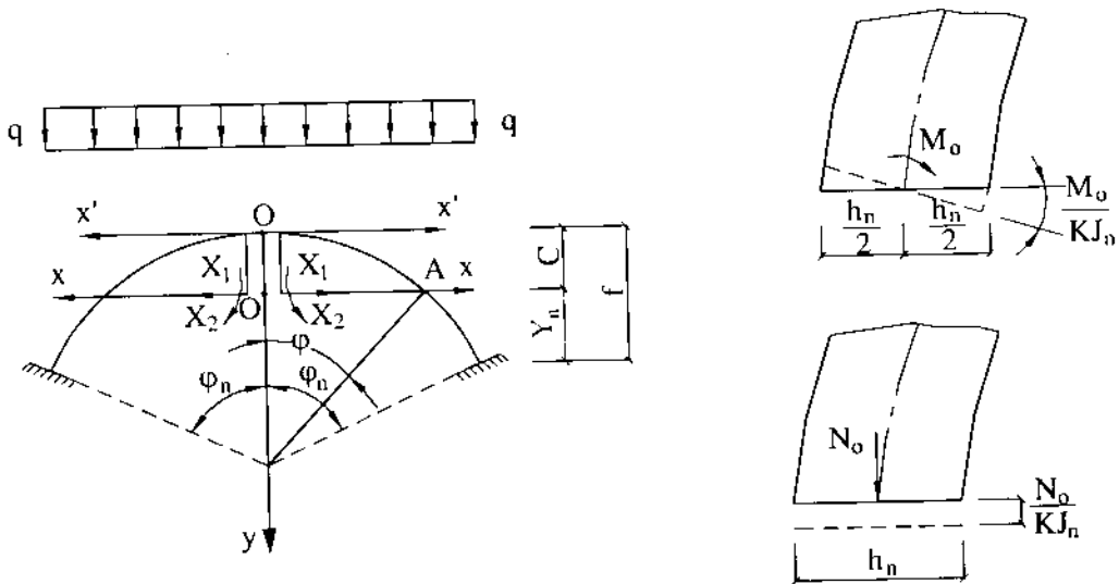
Hình 15-17. Sơ đồ tính toán vòm thấp
