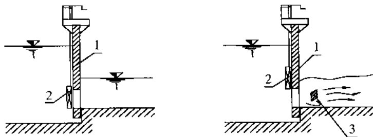
Hình 19-30 : Hệ thống đưa nước tập trung qua cửa van chính.
