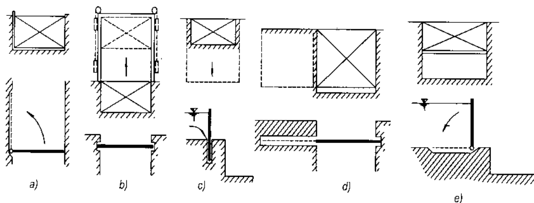
Hình 19-37: Một số hình thức cửa van phẳng.
