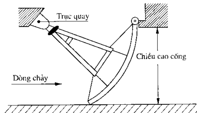
Hình 19-36: Van cung bố trí ngược.
