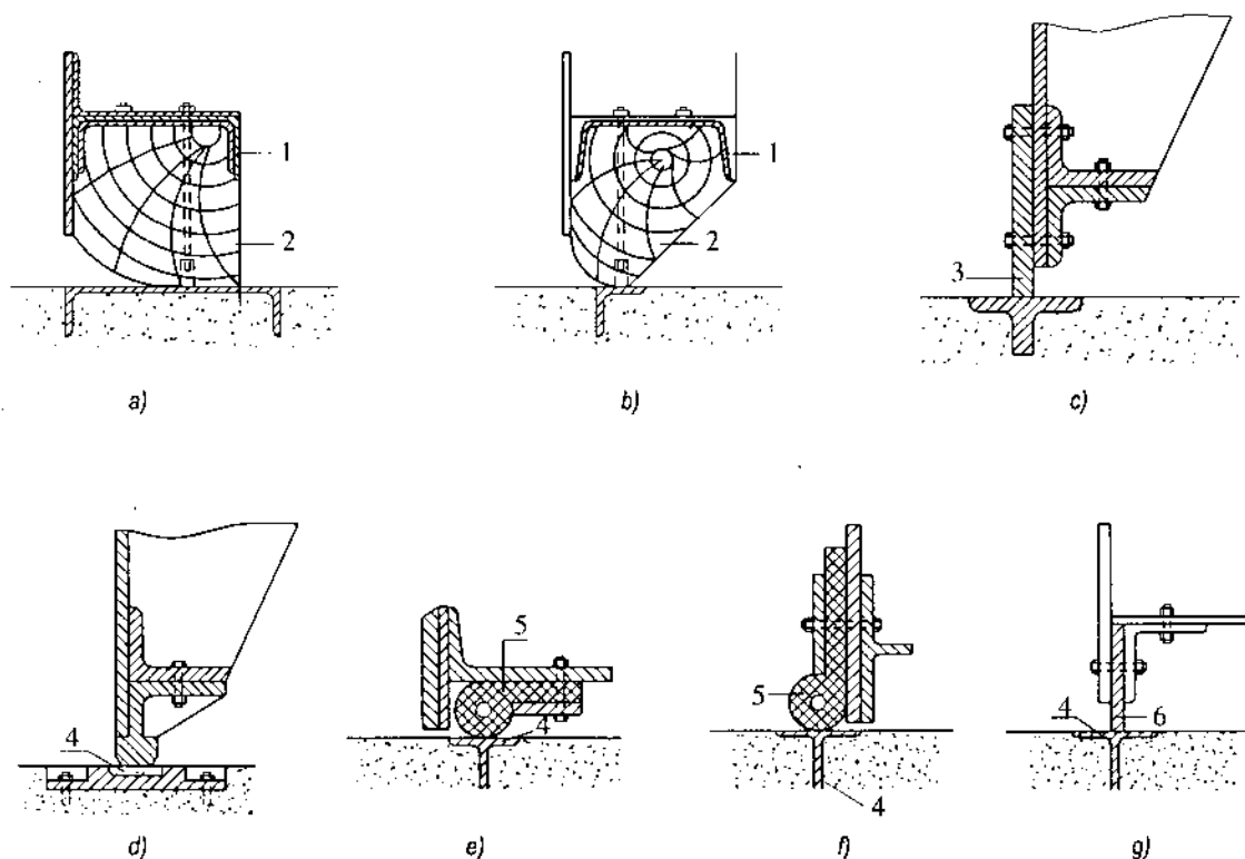
Hình 17-17. Thiết bị chắn nước đáy cửa van phẳng
