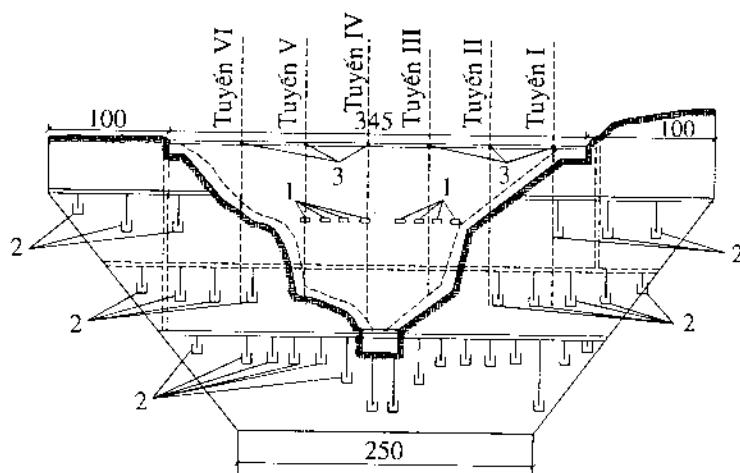
Hình 21-2. Sơ đồ bố trí dụng cụ quan trắc trong đập đất
