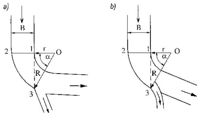
Hình 13-6. Chọn vị trí đặt cửa lấy nước theo N.F.Danheliia
