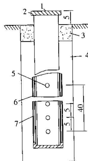
Hình 22-1. Cấu tạo ống đo áp 1.2. Nắp đáy; 3. Lớp bê tông; 4. Cát sỏi; 5. Lỗ; 6. Vải bọc; 7. Lưới thép
