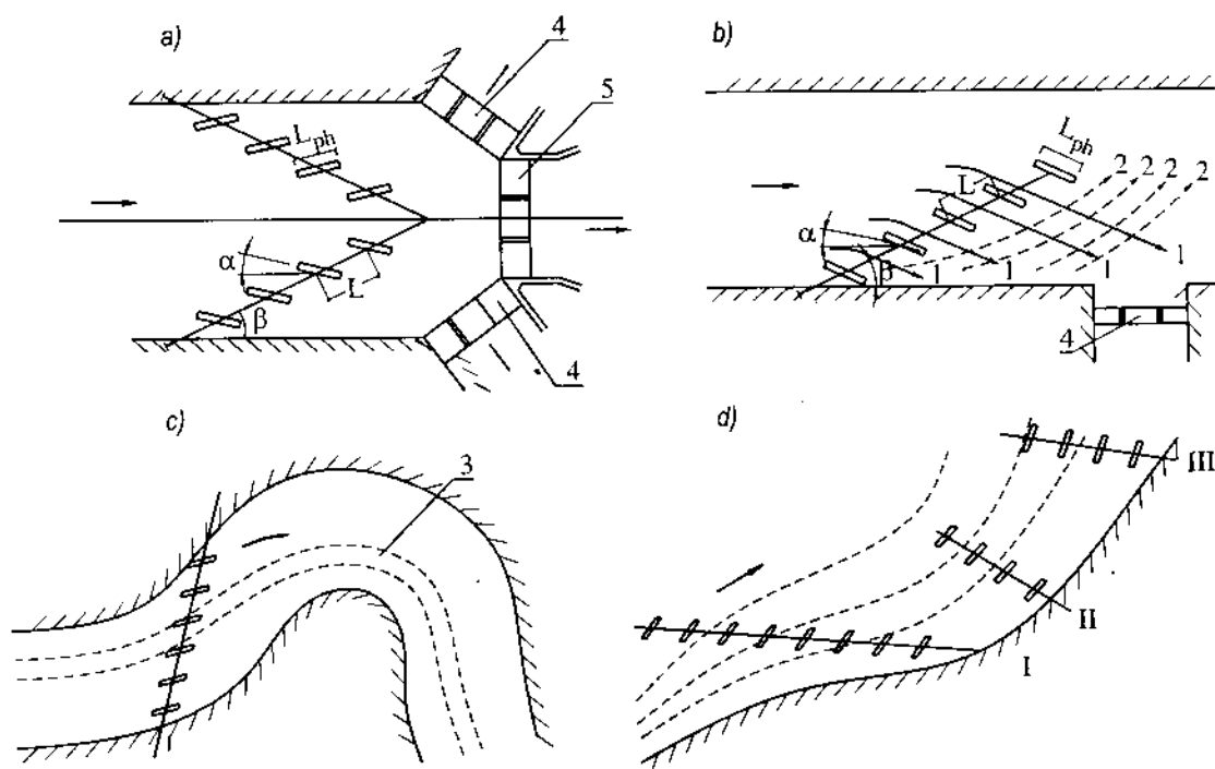
Hình 13-25: Hệ thống lái dòng M.V.Pôtapốp
