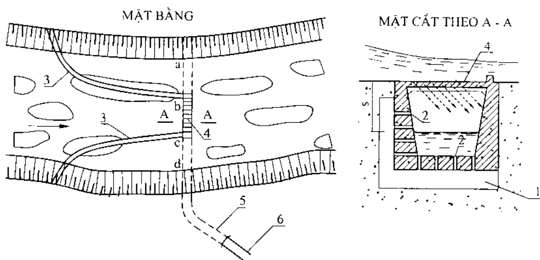
Hình 13-22: Hình thức lấy nước kiểu Kapkaz
