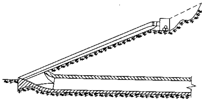
Hình 15-29. Cửa lấy nước kiểu mái nghiêng
