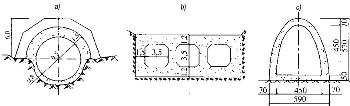
Hình 15-36. Các hình thức mặt cắt cống ngầm
