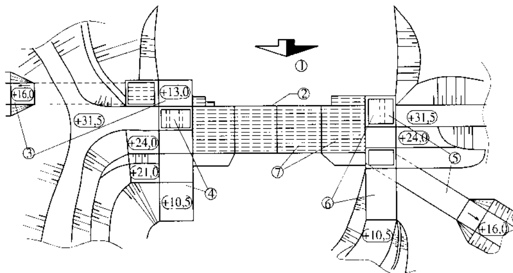
Hình 13-14. Sơ đồ mặt bằng tổng thể đầu mối công trình lấy nước Thạch Nham.
