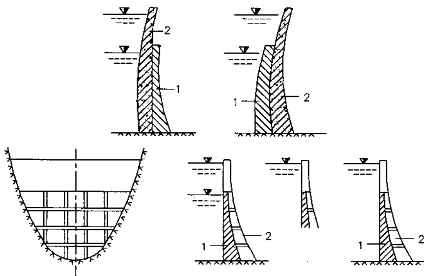
Hình 21-8. Giải pháp tôn cao và mở rộng đập vòm 1. Khối đập cũ, 2. Khối đập tôn cao, mở rộng
