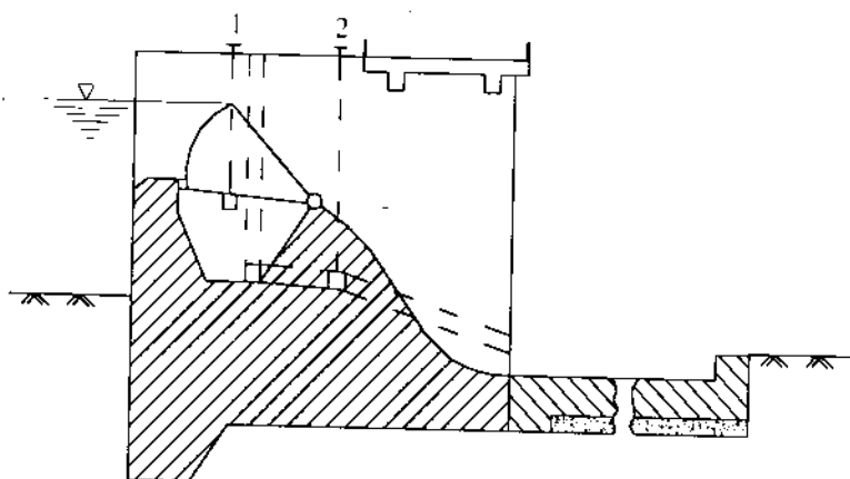
Hình 17-25. Cửa van hình quạt
