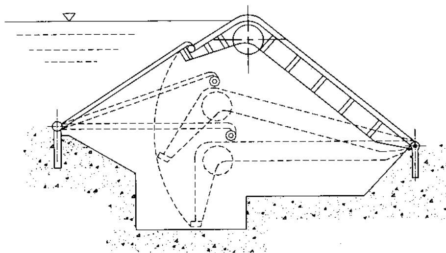
Hình 17-29. Cửa van kiểu mái nhà
