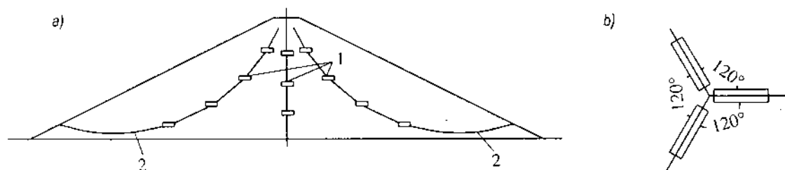
Hình 22-5. Bố trí máy đo áp lực đất
