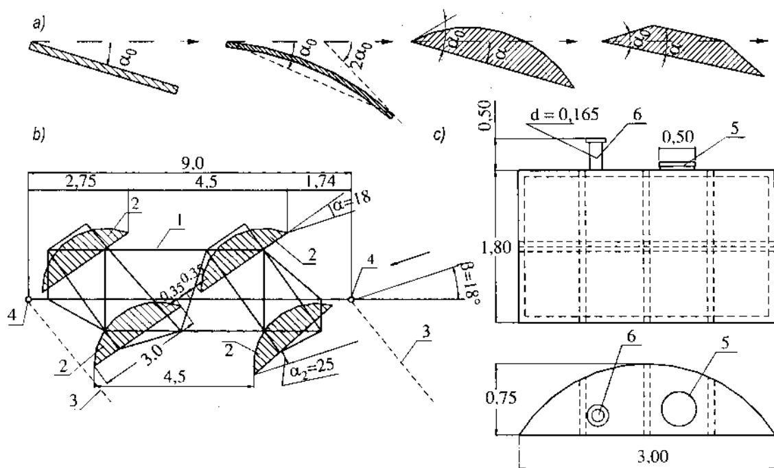
Hình 13-26. Kết cấu của hệ thống lái dòng
