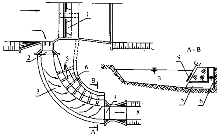
Hình 18-8: Bể lắng cát xối rửa liên tục kiểu L.N.Nikitin
