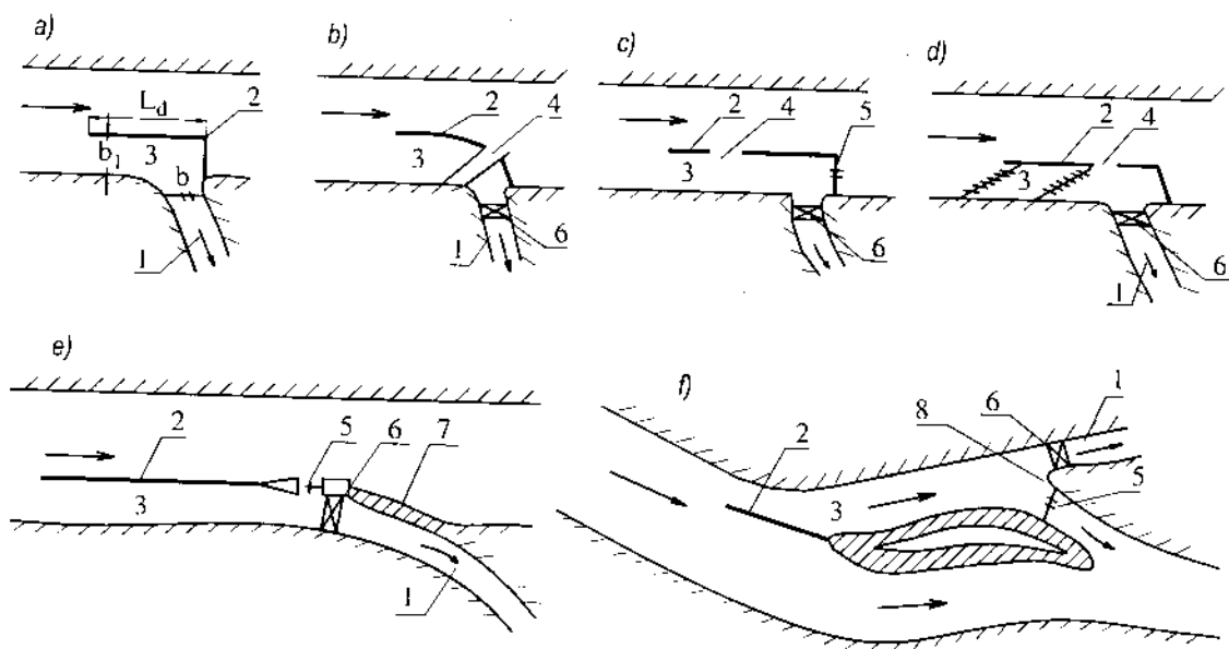
Hình 13-13. Các hình thức lấy nước chính diện không đập.
