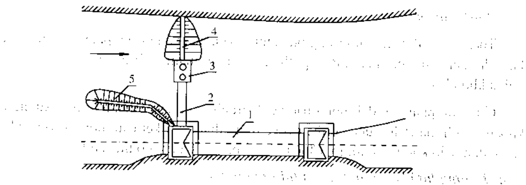
Hình 19-13 : Sơ đồ bố trí âu thuyền trong đầu mối công trình thủy lợi
