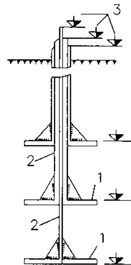
Hình 22-3. Mốc nhiều tầng 1. Tấm; 2. Ống thép; 3. Mốc
