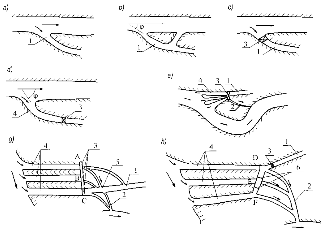
Hình 13-7. Sơ đồ các hình thức lấy nước bên cạnh không đập
