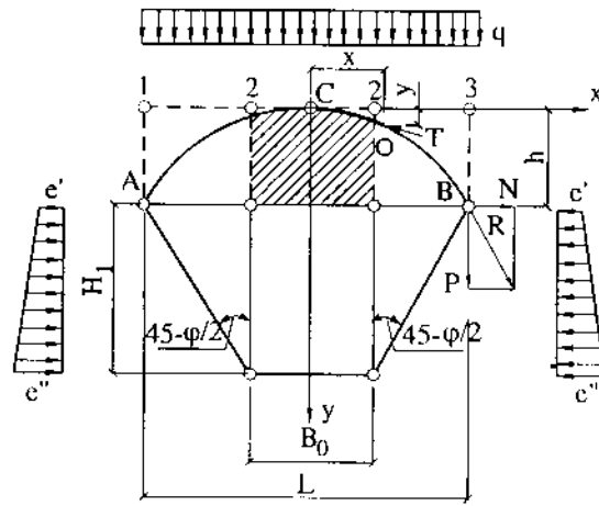
Hình 15-10. Sơ đồ tính áp lực đá núi
