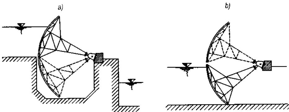
Hình 19-39: Cửa van hình cung.
