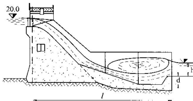
Hình 12-12. Sân tiêu năng có độ dốc thuận
