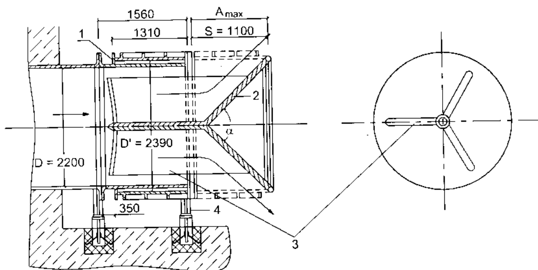
Hình 17-34. Van côn có đường kính 2200mm (đơn vị trong hình vẽ: mm)
