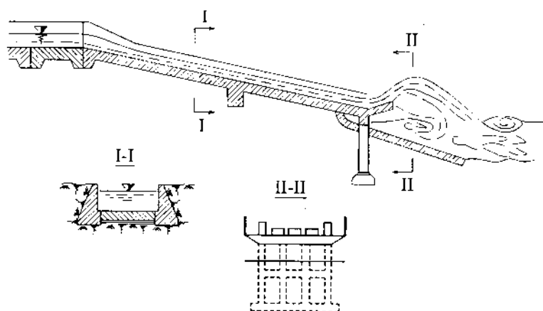
Hình 12-28. Tiêu năng kiểu máng phun
