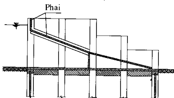
Hình 19-44 : Máng có tấm phai xếp nghiêng.
