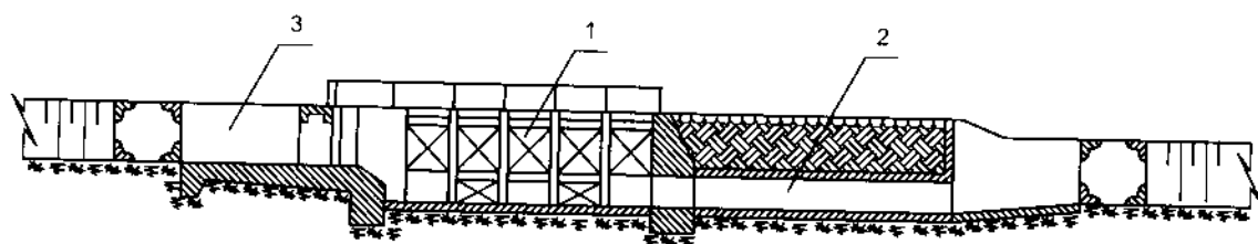
Hình 16-10. Cống trên kênh dẫn nước
