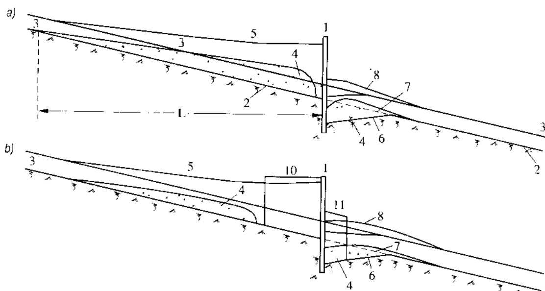
Hình 13-15. Mặt cắt dọc sông vùng đập
