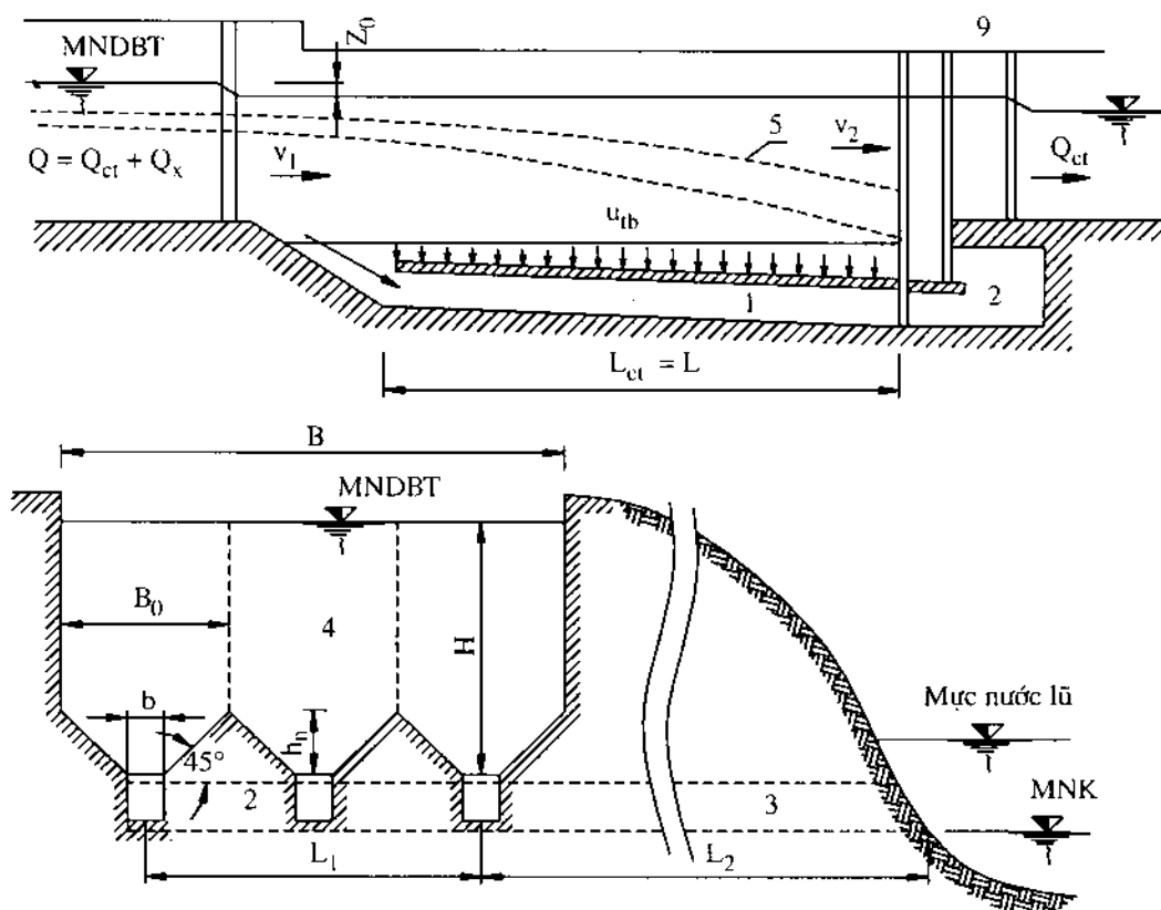
Hình 18-11. Sơ đồ tính toán bể lắng cát xói rửa liên tục.
