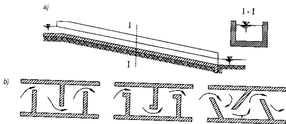
Hình 19-48 : Một số dạng đường cá đi kiểu máng.
