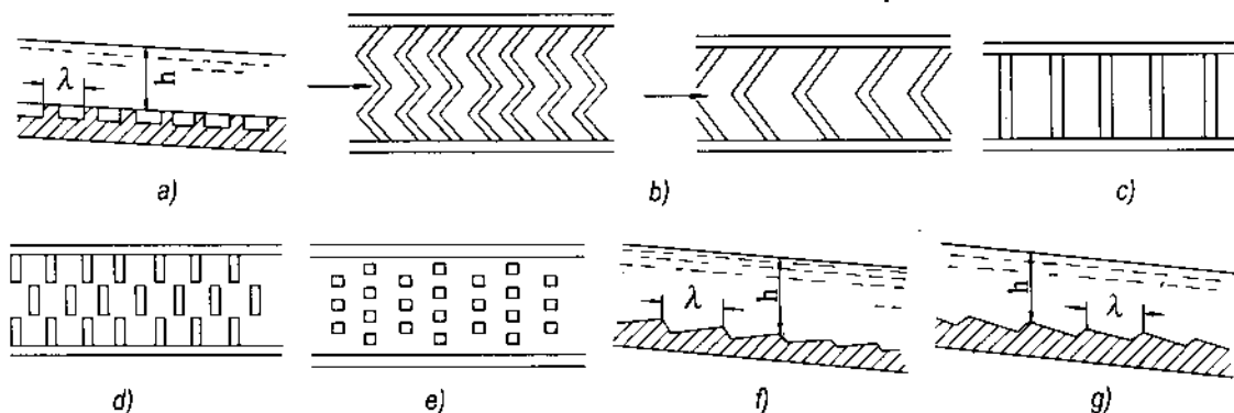
Hình 12-27. Các loại mố nhám nhân tạo
