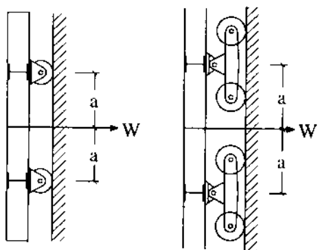
Hình 17-6. Cửa van phẳng có bánh xe lăn
