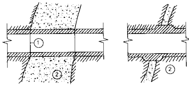
Hình 15-27. Xả lý khi đường hầm xuyên qua các tầng gãy 1. Khe co giãn; 2. Tầng gãy
