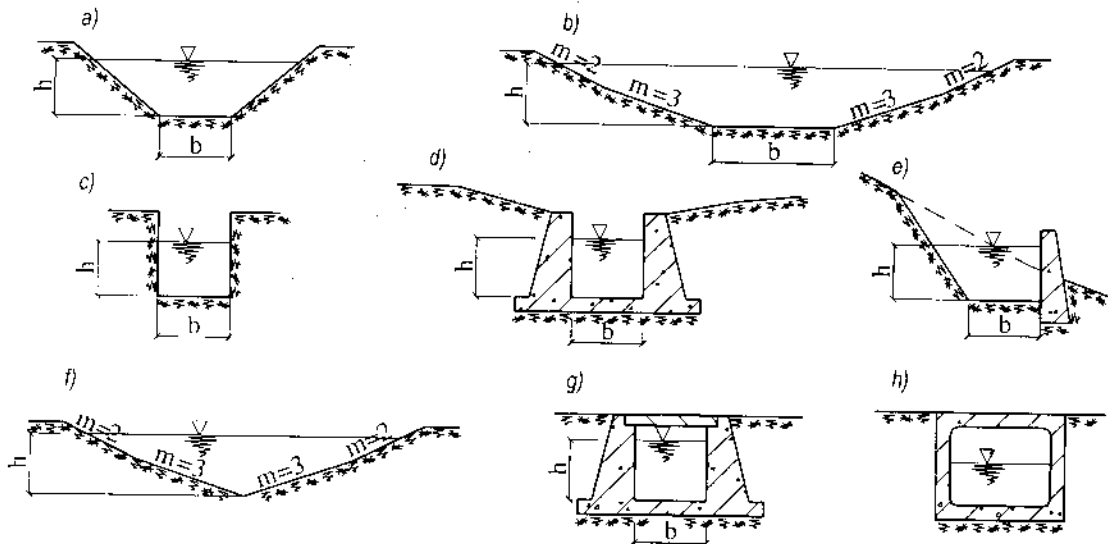
Hình 16-1. Một số hình dạng mặt cắt kênh
