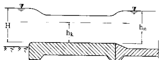
Hình 14-8. Sơ đồ tính thủy lực đập tràn đỉnh rộng.
