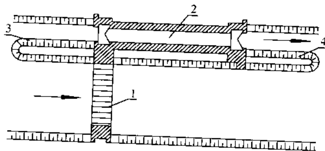
Hình 19-15: Âu thuyền bố trí lùi về phía sau tuyến đập
