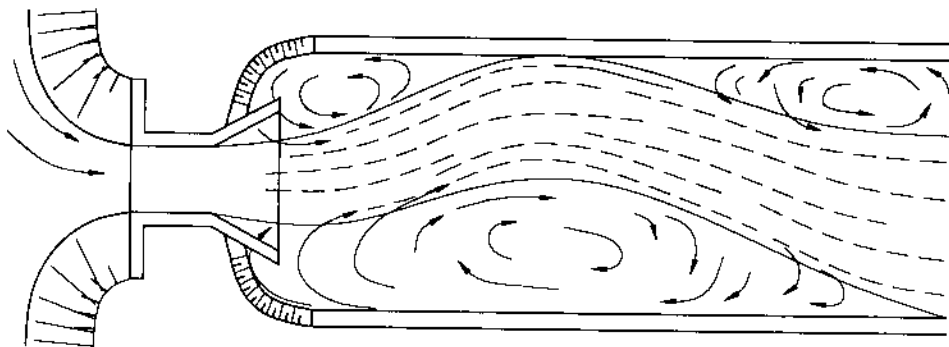
Hình 14-18. Dòng chảy ngoằn ngoèo sau cống.
