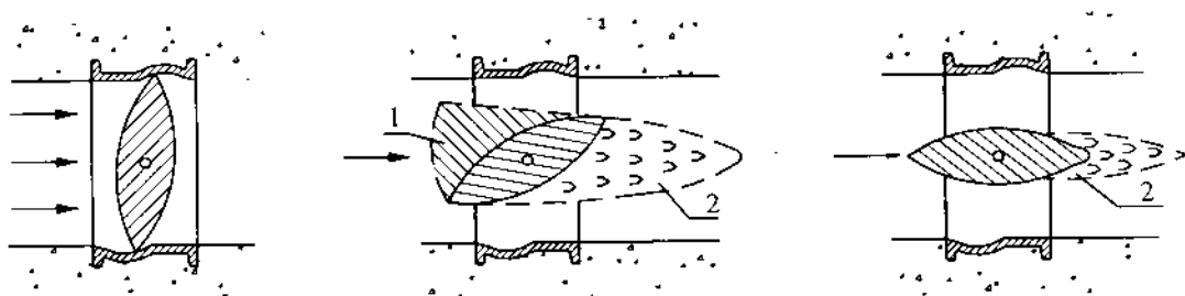
Hình 17-31. Cửa van đĩa trục ngang 1. Khu áp lực dư; 2. Khu nước xoáy.
