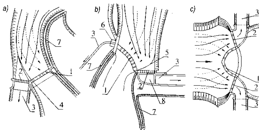
Hình 13-21. Hình thức lấy nước chính diện, bùn cát được xả qua đập tràn.
