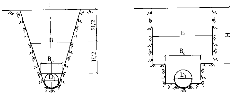
Hình 15-46. Ống chôn trong hào
