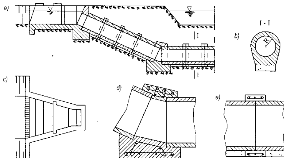
Hình 16-27. Ống xi phông bê tông cốt thép
