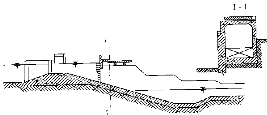
Hình 19-43: Đường thả bè kiểu có buồng.
