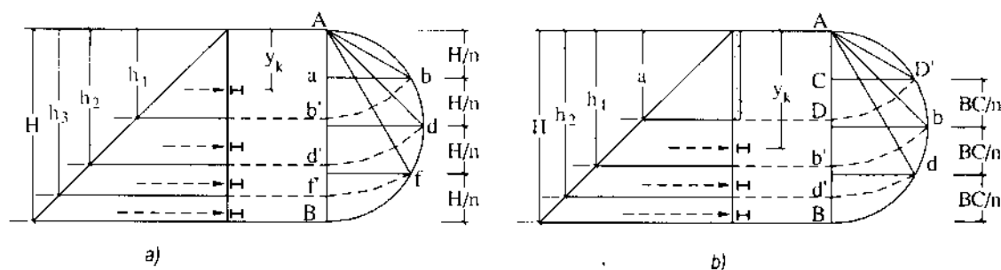
Hình 17-10. Sơ đồ xác định vị trí dầm chính của cửa van phẳng
