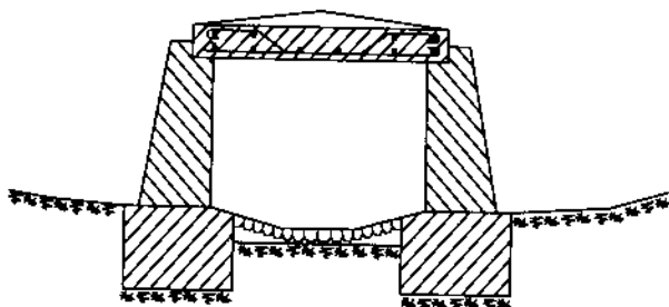
Hình 16-11. Cống ngầm kiểu có tấm nắp
