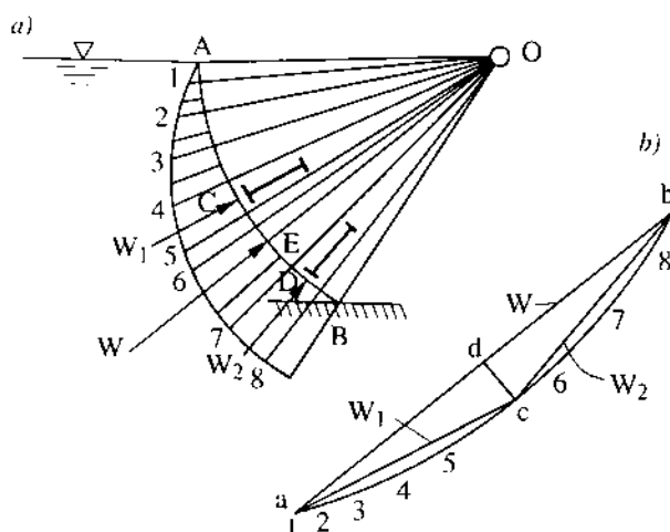
Hình 17-22. Sơ đồ xác định vị trí của dầm chính van cung
