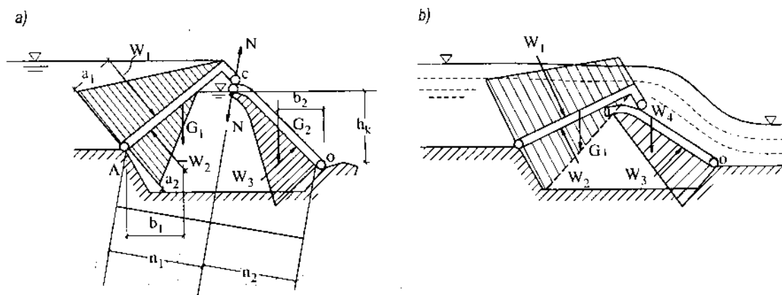
Hình 17-30. Phân tích lực tác dụng lên cửa van mái nhà
