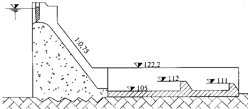
Hình 12-7. Tường tiêu năng
