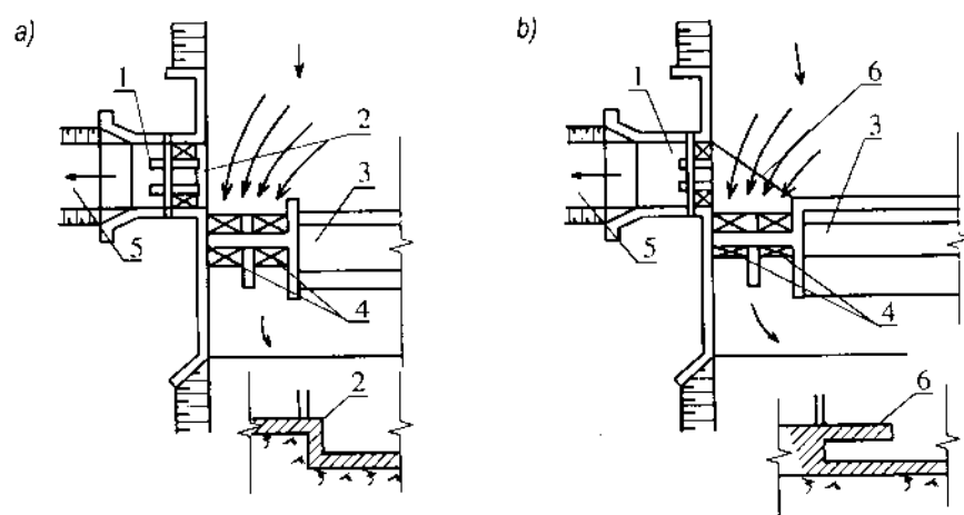
Hình 13-16: Hình thức lấy nước bên cạnh, bùn cát xả qua lỗ đặt ở thân đập
