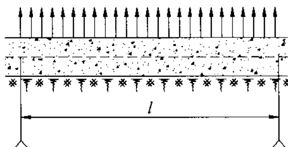
Hình 12-19. Sơ đồ lực và bố trí thép néo trên sân sau
