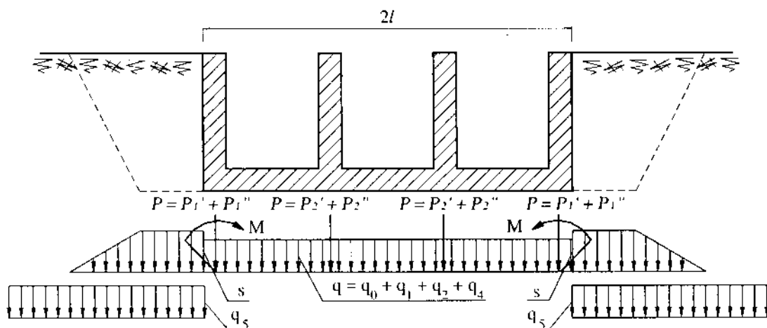
Hình 14-21. Sơ đồ phân tích lực tác dụng lên bản dầm
