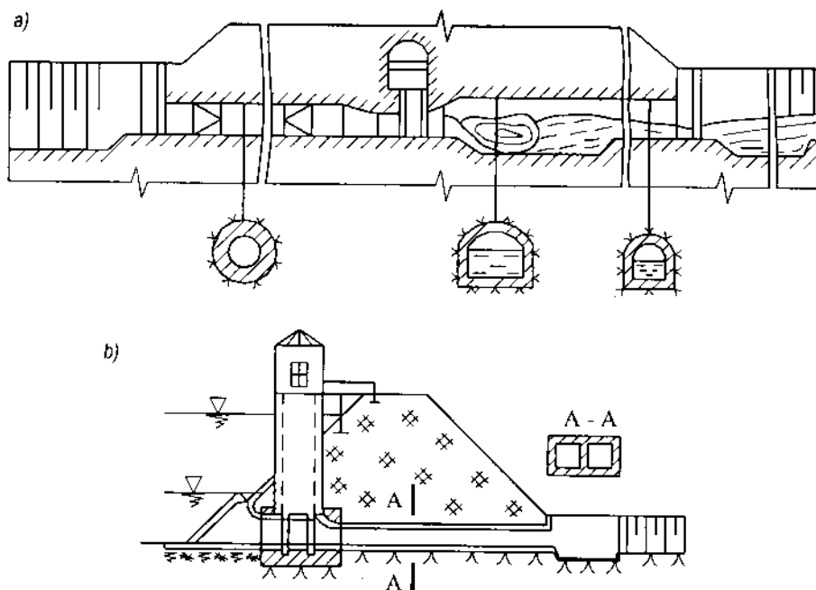
Hình 15-1. a) Đường hầm; b) Cống ngầm
