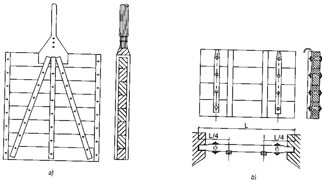
Hình 17-12. Cửa van phẳng bằng gỗ
