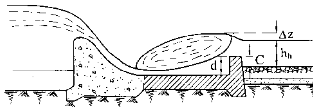
Hình 12-8. Bể và tường tiêu năng kết hợp
