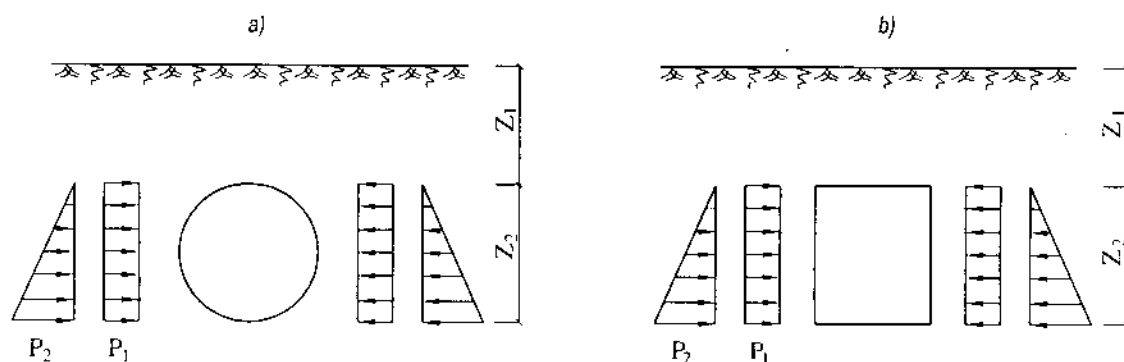
Hình 15-49. Sơ đồ áp lực đất tác dụng lên thành cống
