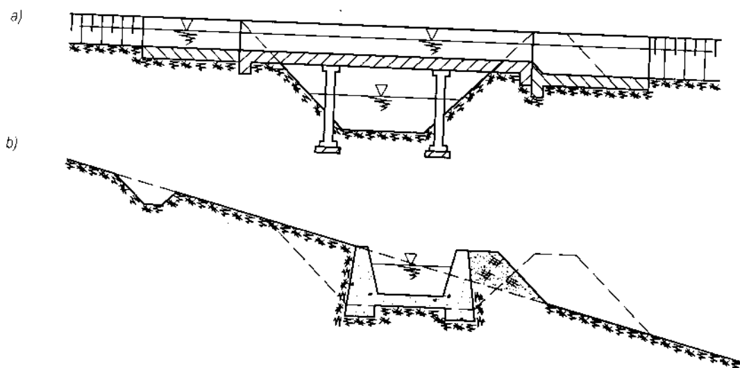
Hình 16-13. a) Cầu máng chuyển nước; b) Kênh xây có vai trò như cầu máng
