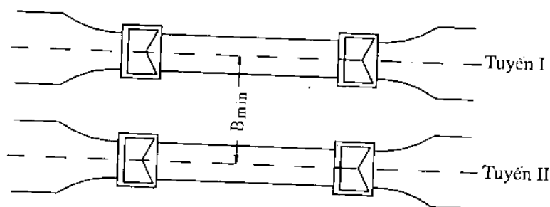
Hình 19-12: Bố trí âu thuyền trong kênh và sự phát triển trong tương lai
