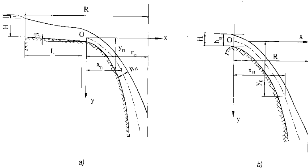
Hình 12-38. Hình dạng loa tràn a) Ngưỡng có mặt phẳng nghiêng; b) Ngưỡng không có mặt phẳng nghiêng.
