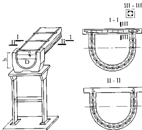
Hình 16-22. Sơ đồ cầu máng vỏ mỏng
