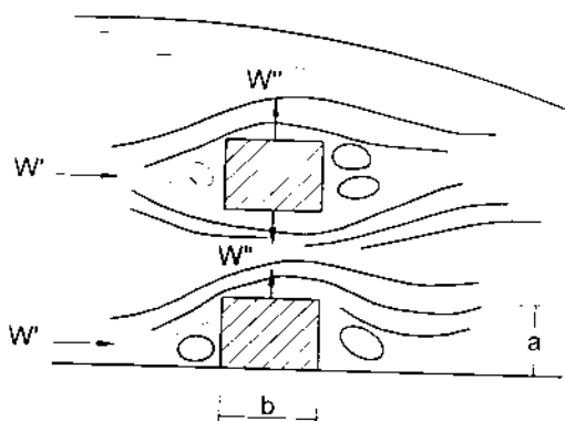
Hình 17-14. Sơ đồ lực thủy động tác dụng lên dầm phai
