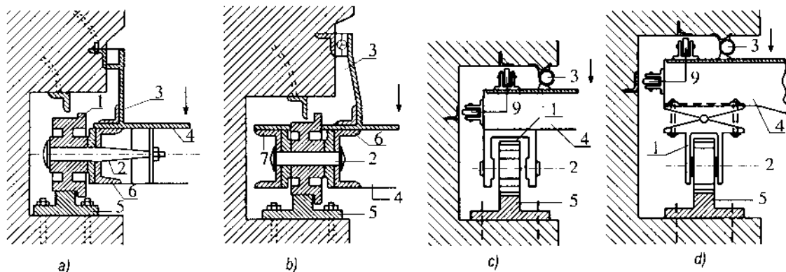
Hình 17-16. Một số hình thức bánh xe cửa van phẳng
