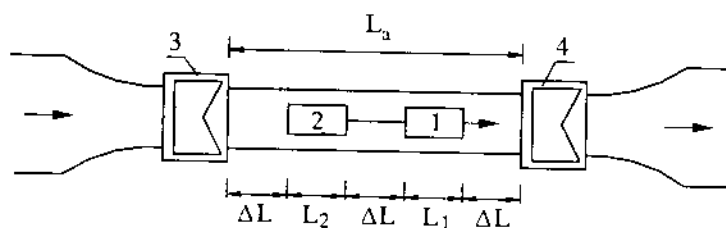
Hình 19-18: Sơ đồ tính toán chiều dài buồng âu 1. Tàu kéo; 2. Thuyền; 3 và 4. Đầu âu thượng và đầu âu hạ
