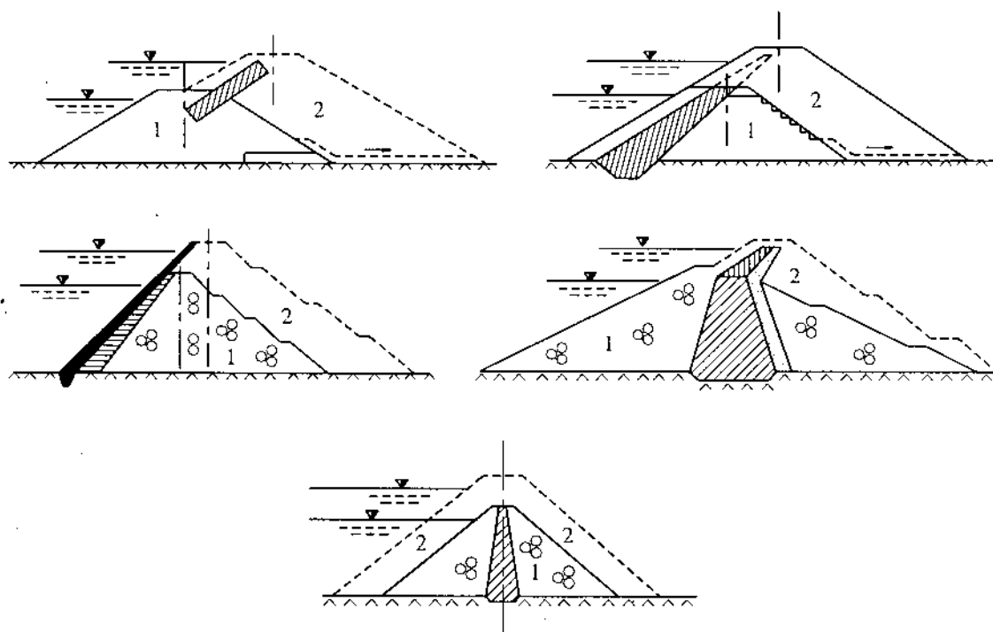
Hình 21-5. Một số giải pháp tôn cao và mở rộng đập bằng vật liệu địa phương 1. Khối đập cũ, 2. Khối đập tôn cao, mở rộng
