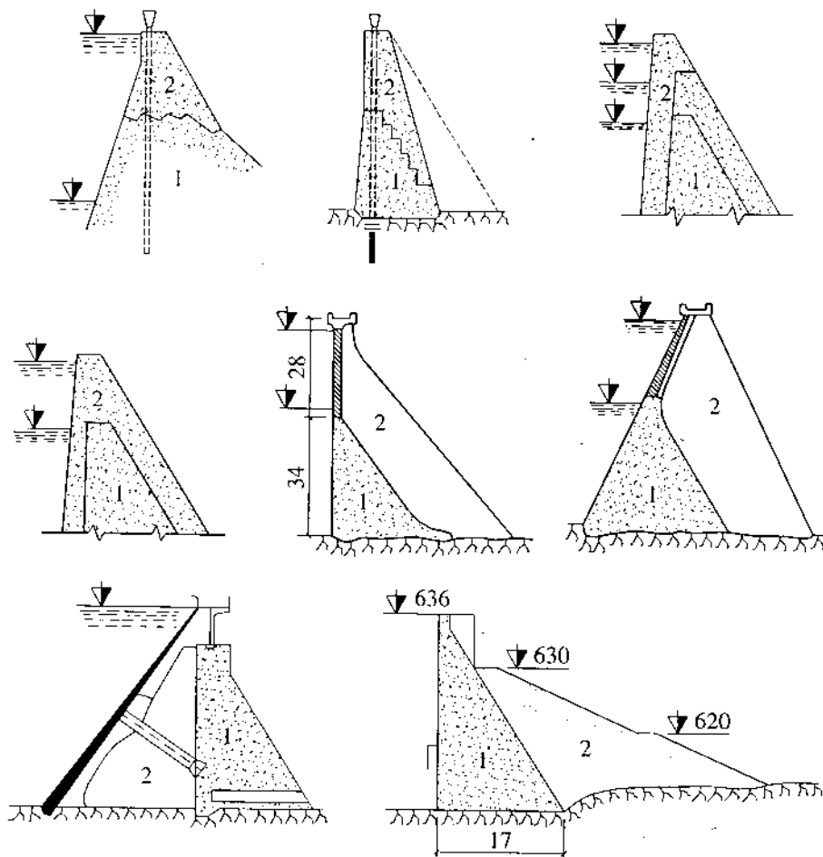
Hình 21-6. Một số giải pháp tôn cao và mở rộng đập bê tông trọng lực 1. Khối đập cũ, 2. Khối đập tôn cao, mở rộng
