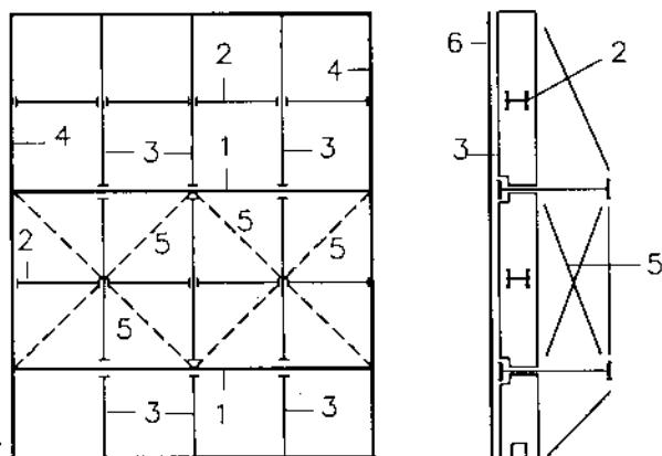
Hình 17-8. Hệ thống dầm và bản của cửa van phẳng
