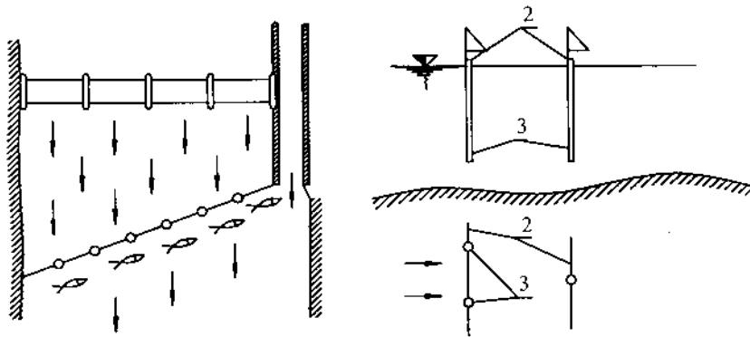
Hình 19-47: Bố trí lưới chắn cá. 1. Lưới; 2. Dây cáp; 3. Cực điện
