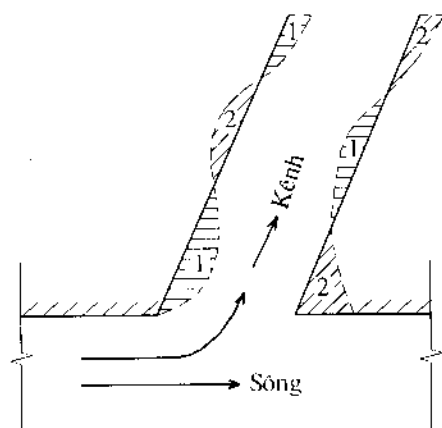
Hình 13-5. Cửa lấy nước ở bờ không ổn định 1. Vùng bồi lắng; 2. Vùng xói lở.
