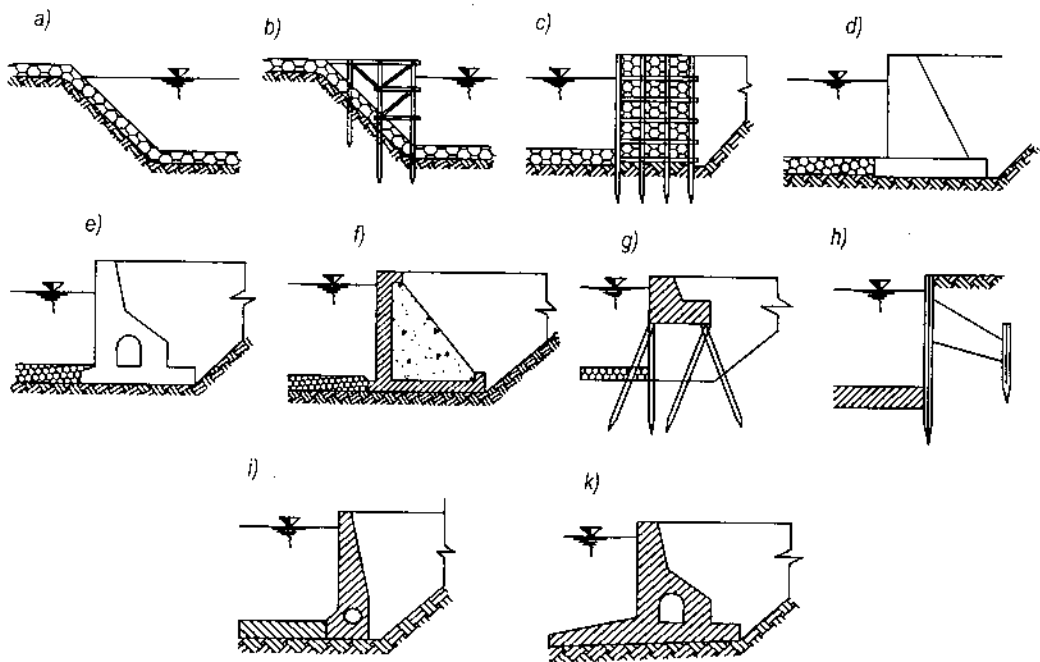
Hình 19-27: Một số hình thức mặt cắt ngang buồng âu thuyền
