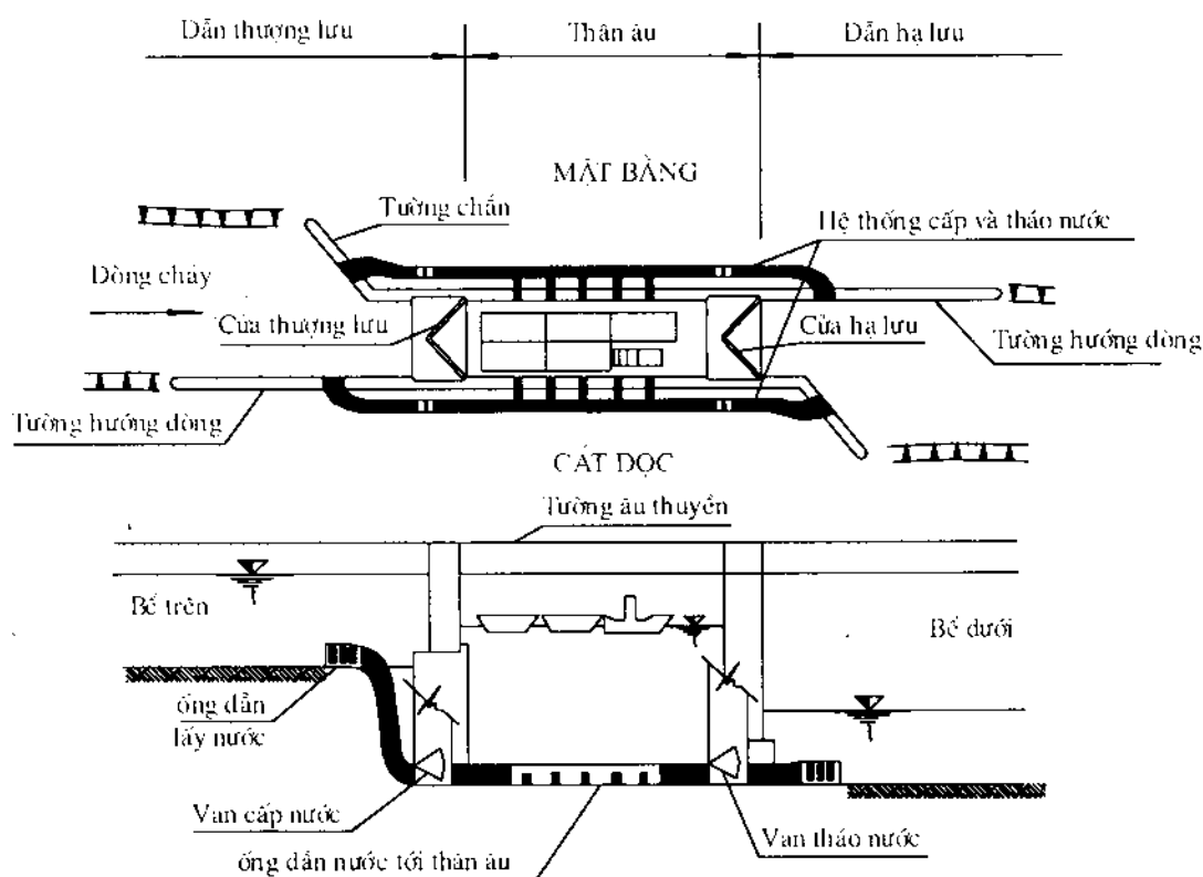
Hình 19-3: Bố trí chung âu thuyền có các cống dẫn nước đặt trong tường bên
