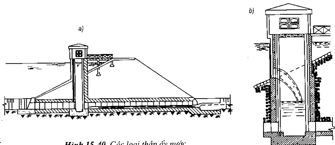
Hình 15-40. Các loại tháp lấy nước
