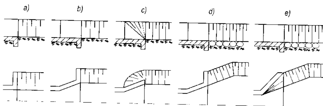
Hình 14-32. Một số loại tường cánh hạ lưu.
