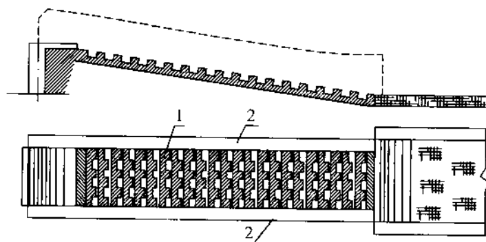
Hình 19-42: Máng thả bè có mố nhám đáy 1. Mố nhám; 2. Tường chắn.
