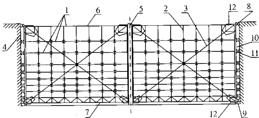
Hình 19-40: Các bộ phận của cửa van chữ V
