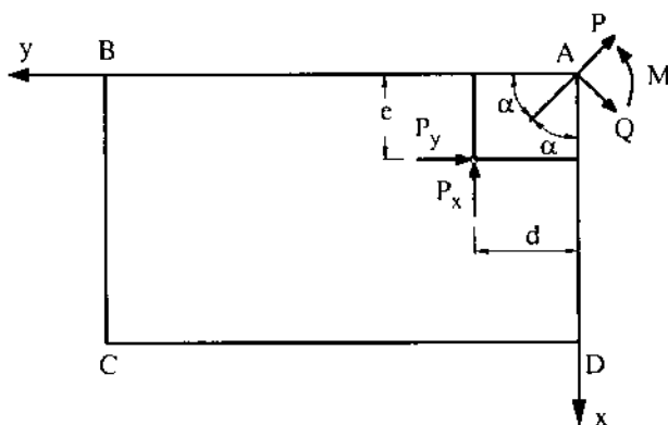
Hình 14-27. Sơ đồ tính toán trụ van cung.
