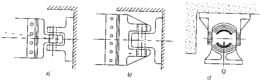
Hình 17-23. Khớp quay của cửa van còng a, b) Khớp trụ; c) Khớp cầu
