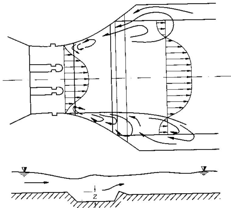
Hình 14-15. Dòng chảy khi nhảy sóng
