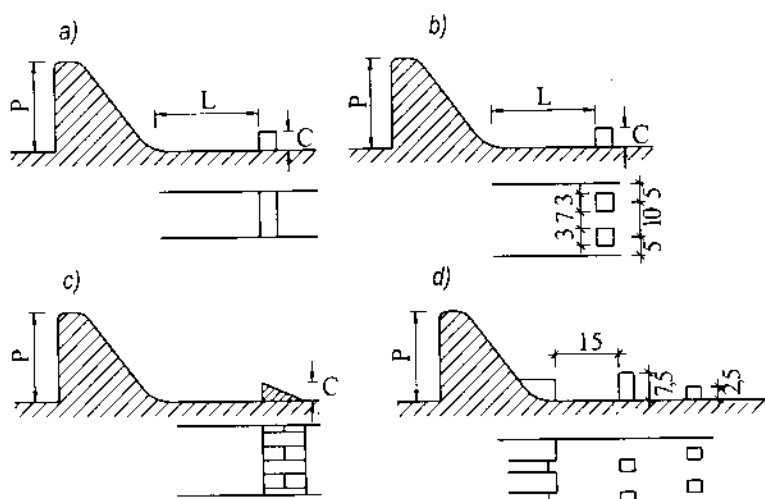
Hình 12-9. Hình thức các thiết bị tiêu năng (kích thước trong hình ghi theo m)
