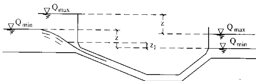
Hình 16-24. Sơ đồ tính toán thủy lực xi phông ngược
