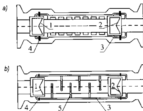
Hình 19-34: Sơ đồ dẫn tháo nước kiểu phân tán.
