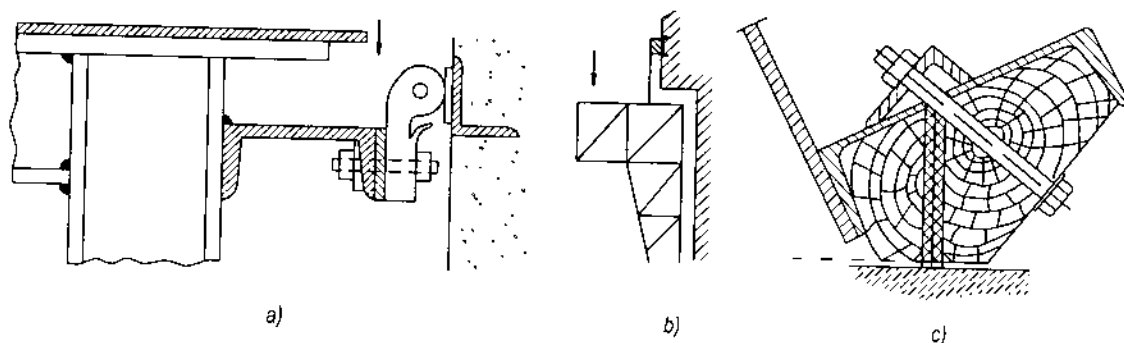
Hình 17-24. Một số thiết bị chặn nước của van cung a, b) Chặn nước bên cạnh; c) Chặn nước đáy.
