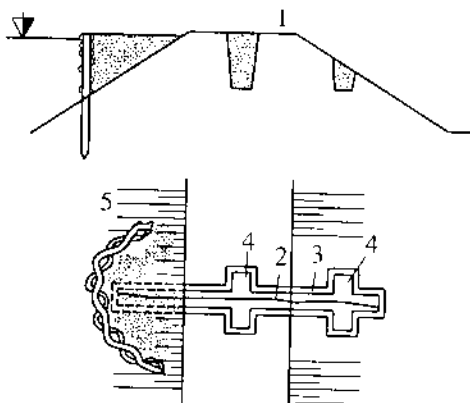
Hình 21-3. Xử lý khe nứt đắp đất thẳng góc với trục đập 1. Đỉnh đập, 2. Vết nứt, 3. Rãnh đào, 4. Rãnh nêm, 5. Đê quay
