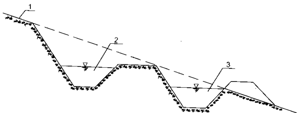
Hình 16-7. Sơ đồ bố trí kênh tiêu sườn dốc 1. Sườn dốc; 2. Kênh tiêu; 3. Kênh dẫn
