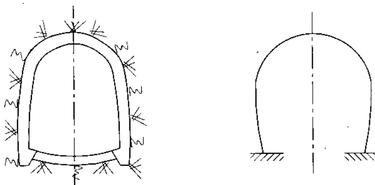
Hình 15-18. Sơ đồ tính toán vòm cao
