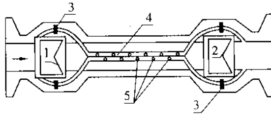
Hình 19-35 : Hệ thống dẫn nước kiểu phân tán ở đáy. 1 và 2. Cửa van đầu âu thượng và hạ; 3. Van đường dẫn tháo nước; 4. Ống dẫn tháo nước; 5. Các lỗ thoát nước.
