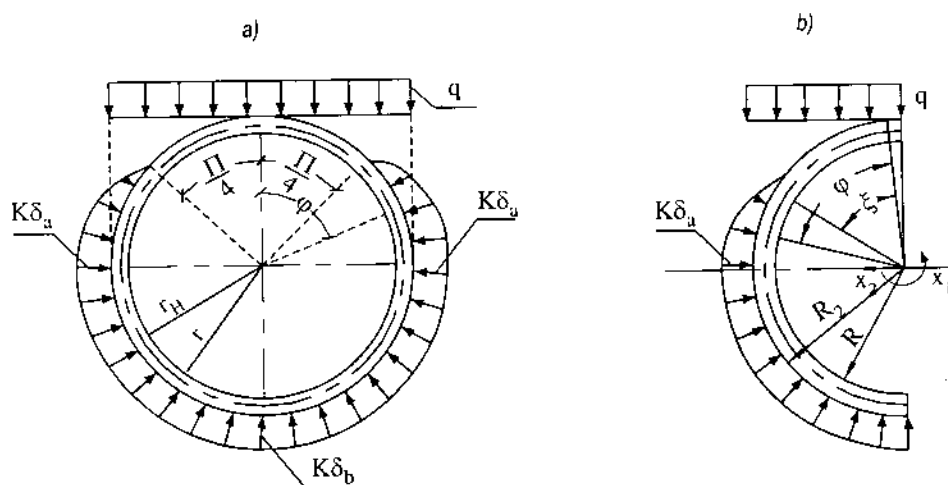
Hình 15-25. Sơ đồ tính toán lớp lót dưới tác dụng của áp lực đá núi thẳng đứng
