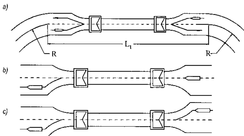
Hình 19-17 : Các hình thức mặt bằng đoạn kênh dẫn.
