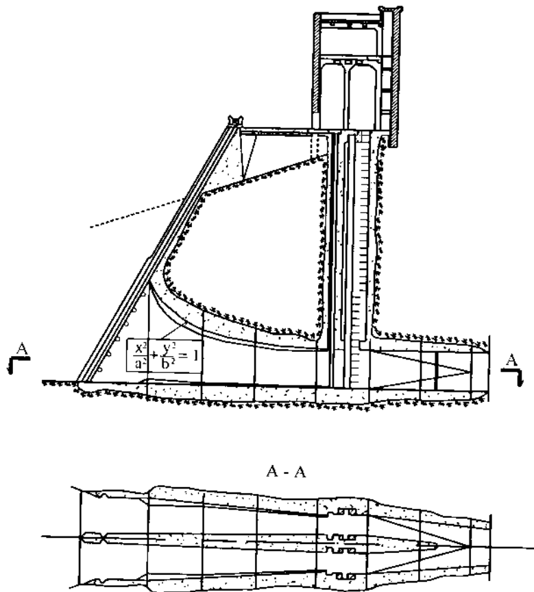
Hình 15-28. Cửa lấy nước kiểu giếng đứng
