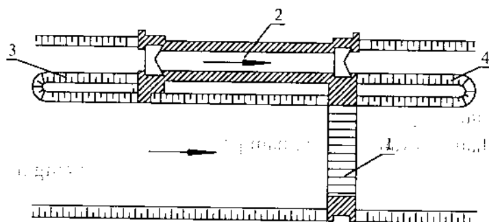
Hình 19-14: Âu thuyền bố trí nhô về phía trước tuyến đập
