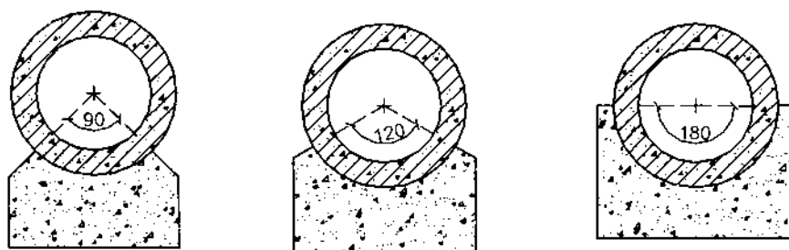
Hình 15-54. Các kiểu bệ đỡ ống ngầm
