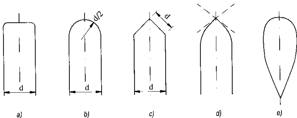
Hình 12-17. Các hình thức trụ pin
