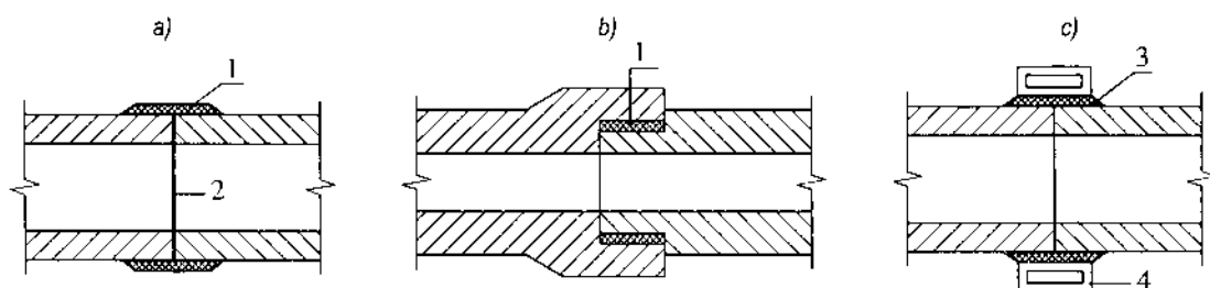
Hình 15-53. Thiết bị chống thấm của các đoạn ống tròn
