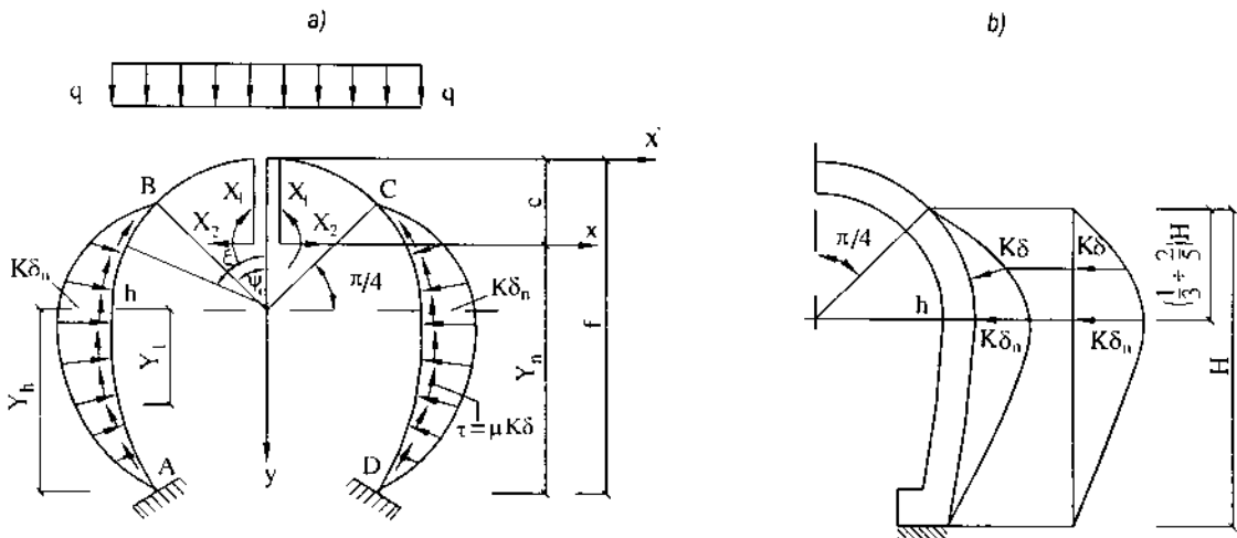
Hình 15-19. a) Sơ đồ tính toán kết cấu vòm cao; b) Xác định vị trí có lực kháng đàn tính lớn nhất trên vòm.
