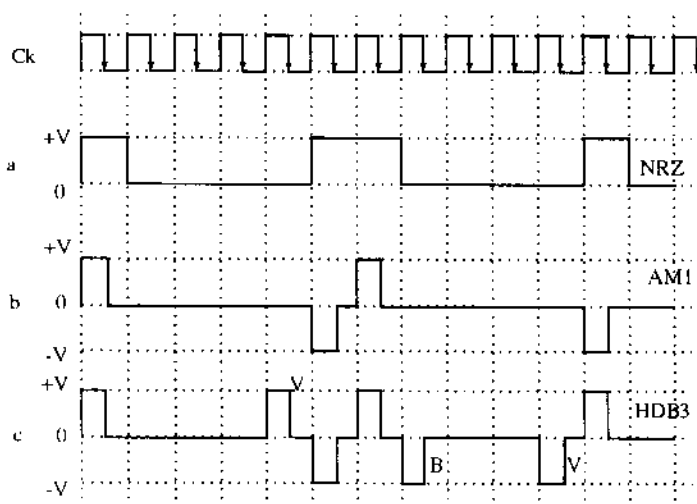
Hình 6.8. Biến đổi mã nhị phân sang mã đường dây
