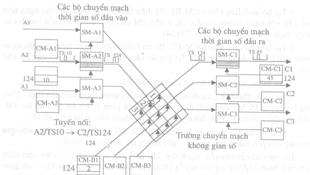
Hình 2.11. Trường chuyển mạch ghép T-S-T
