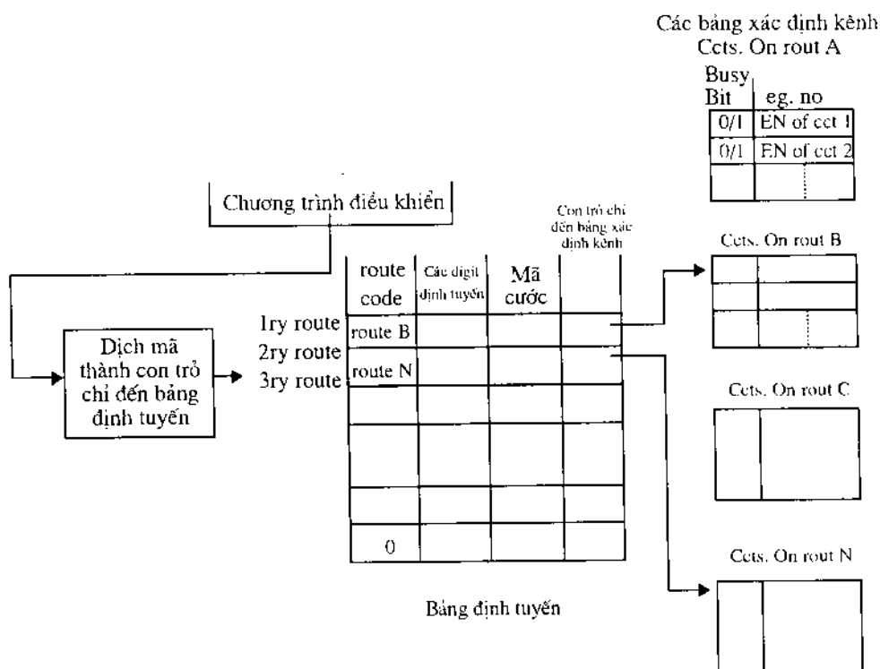
Hình 8.5. Dịch chữ số - Vai trò của các bảng định tuyến
