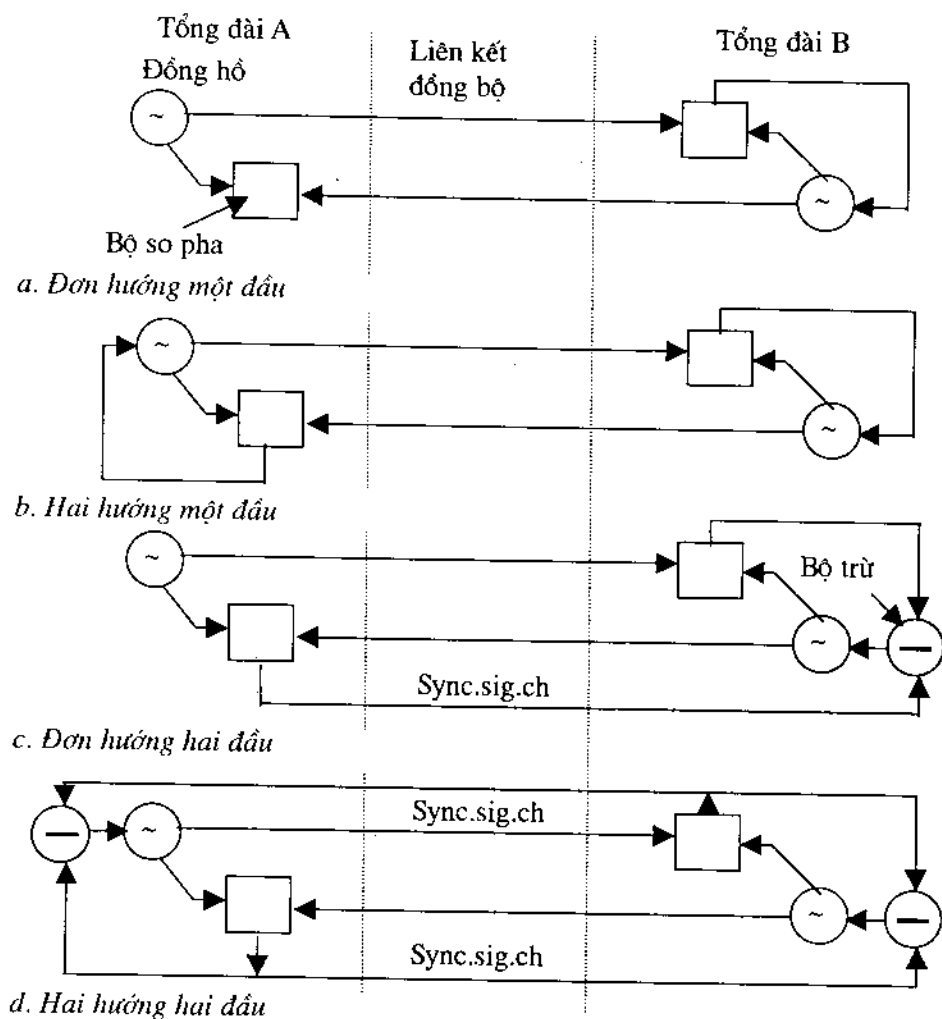
Hình 1.28. Đơn vị đồng hồ của tổng đài kỹ thuật số
