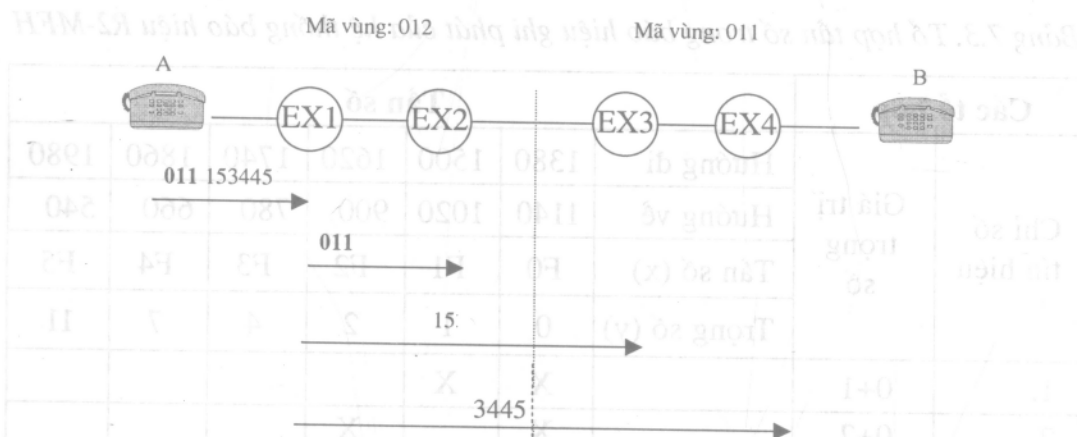
Hình 7.6. Báo hiệu kiểu xuyên suốt (End - To- End)
