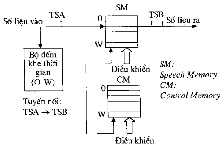
Hình 2.5. Cấu trúc trường chuyển mạch thời gian tín hiệu số
