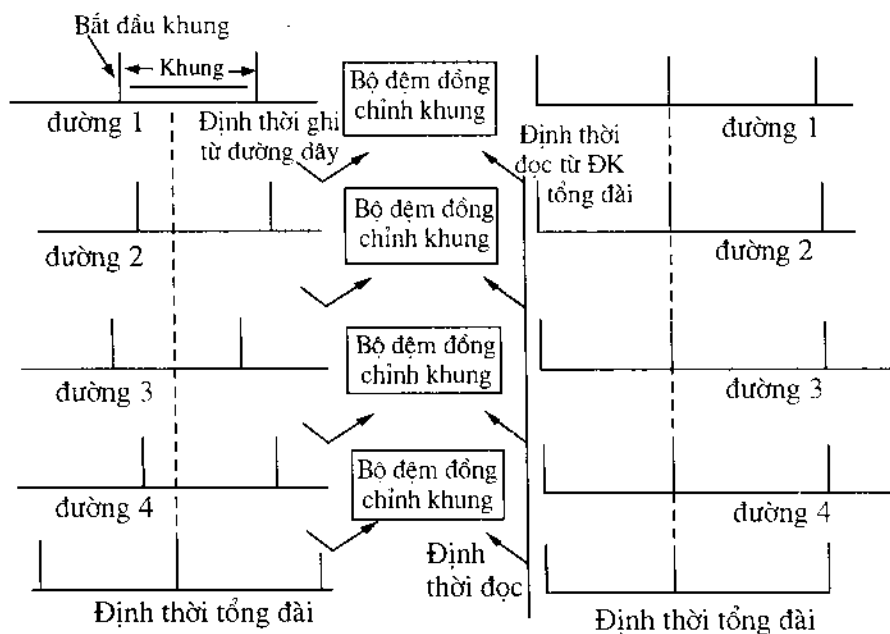
Hình 6.9. Đồng chỉnh khung PCM
