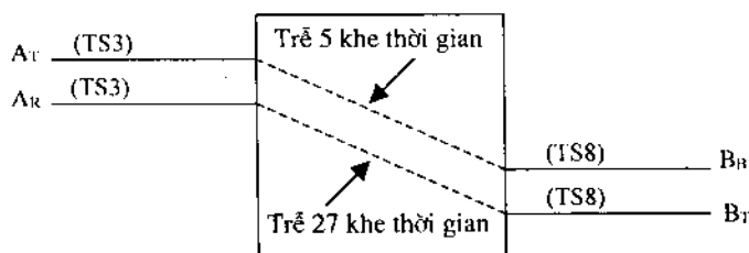
Hình 2.4. Trao đổi khe thời gian
