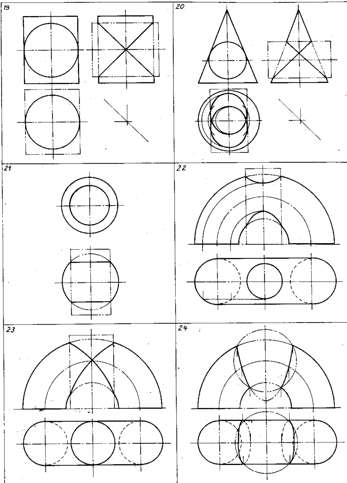
Hình PL 2-3 : Giao tuyến của hai mặt cong. bài : 19 + 24.
